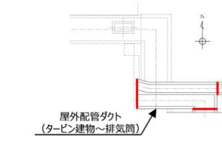
② 屋外配管ダクト (タービン建物〜排気筒) 平面図
