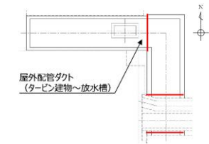
② 屋外配管ダクト (タービン建物〜放水槽) 平面図
