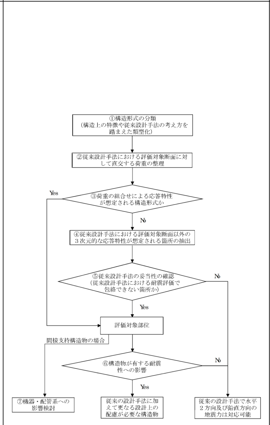
第3.3-3図 水平2方向及び鉛直方向地震力の組合せによる影響 評価のフロー
