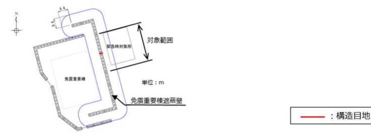
⑤ 免震重要棟遮蔽 平面図
