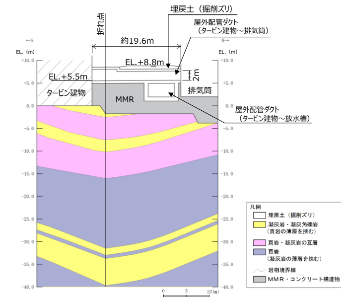
第3.3.5-5図 屋外配管ダクト (タービン建物～排気筒) と屋外配管ダクト (タービン建物～放水槽) との一体化部 断面図 (⑤-⑤断面)
