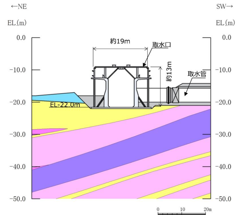
第3.3.5-7図 取水口 断面図 (②-②断面)
