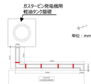
④ 屋外配管ダクト (ガスタービン発電機用軽油タンク基礎〜ガスタービン発電機) 平面図
