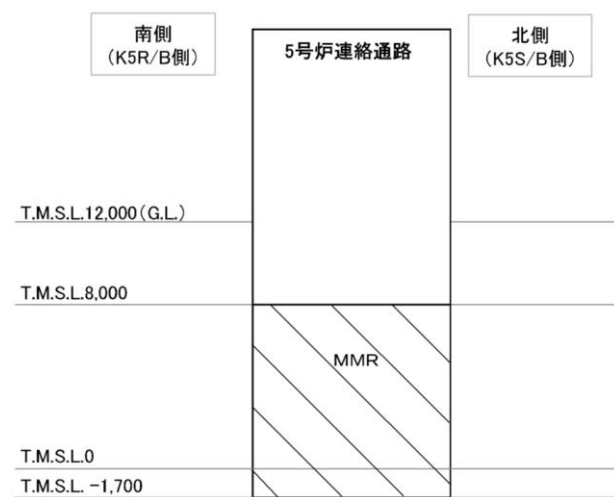
(a) 平面図
