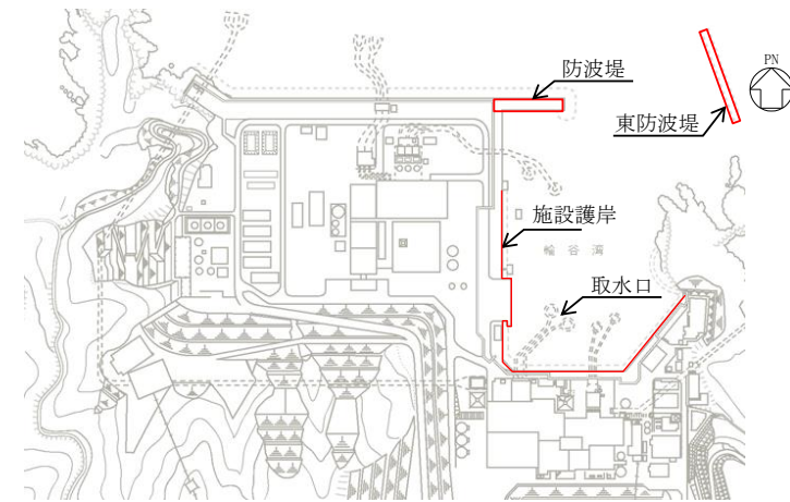
第 2 図 防波堤及び施設護岸の配置
