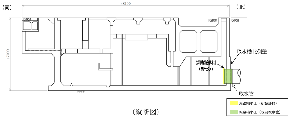
第4.1-8図 1号炉取水槽流路縮小工配置図
