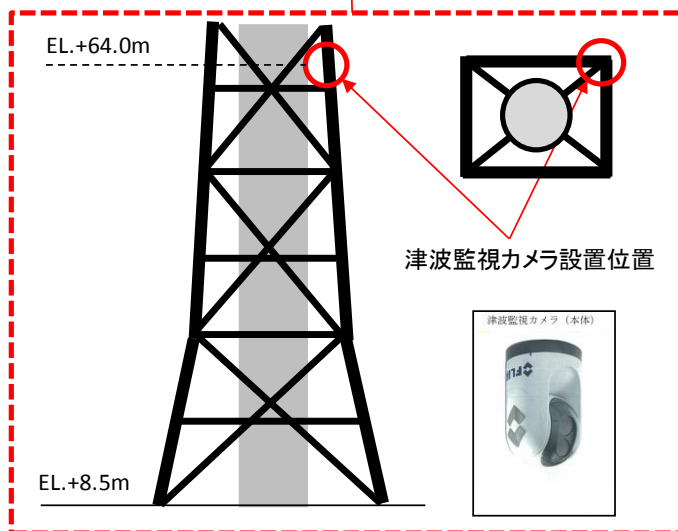
第4.3-2図 津波監視カメラ設置位置
