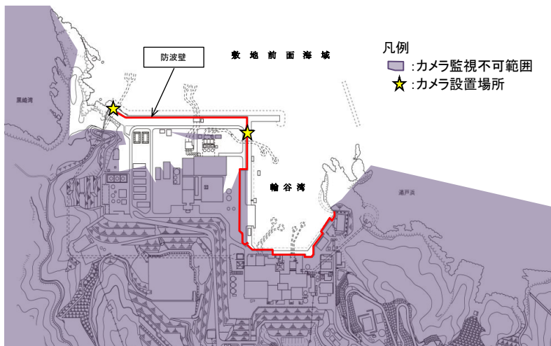
第4.3-5-1図 津波監視カメラが1台機能喪失した場合の視野範囲 (2号炉排気筒E.L.+64.0m位置が機能喪失した場合)
