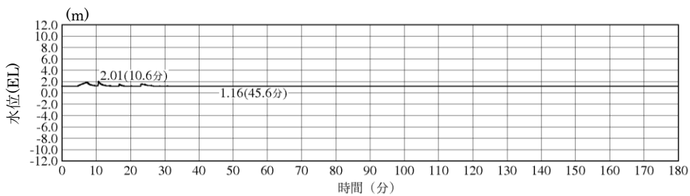
1号炉放水槽（入力津波4，防波堤無し）
