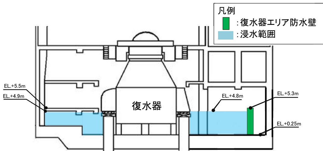
(A-A 断面)
