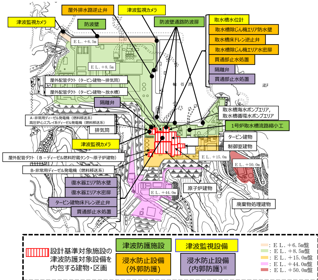
第 2.1-1 図 敷地の特性に応じた津波防護の概要
