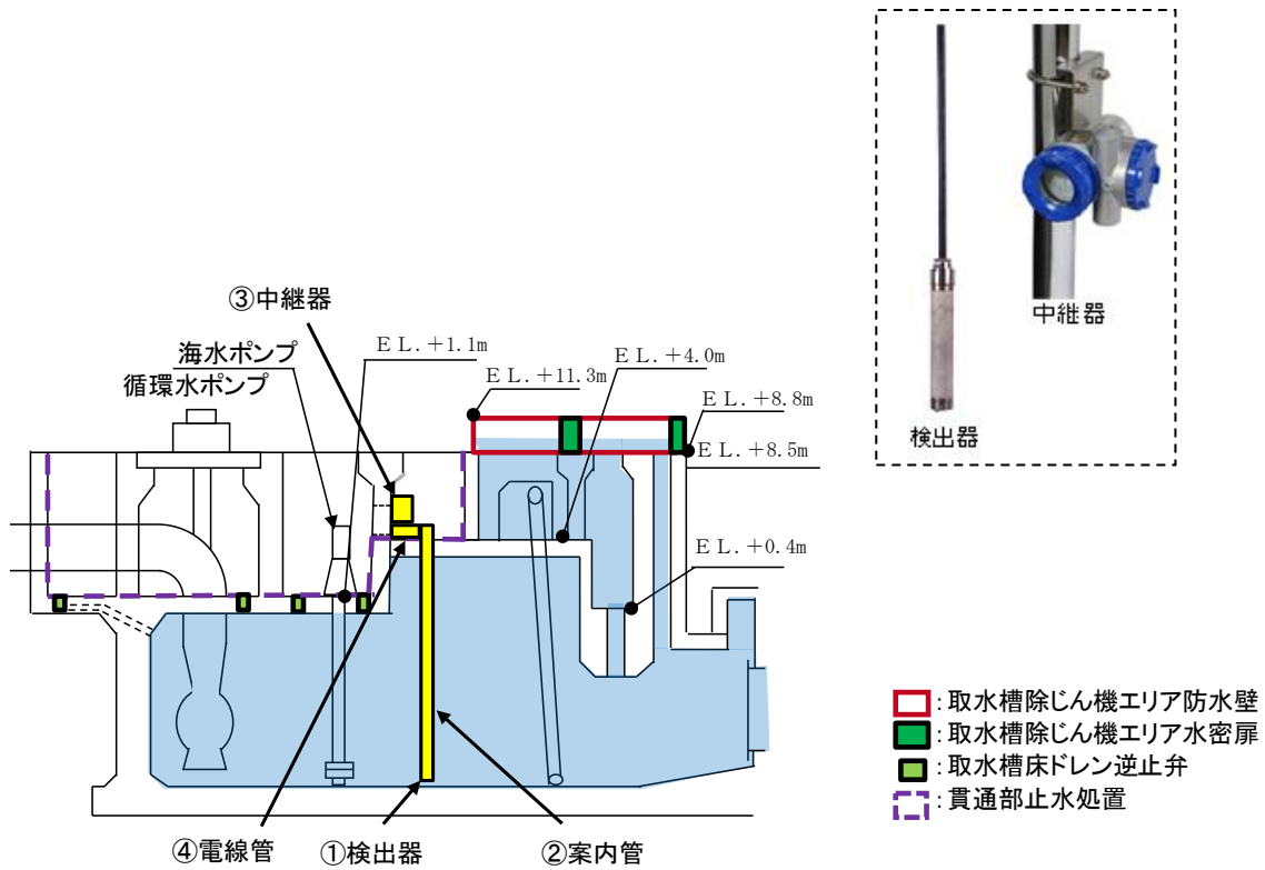
第4.3-10図 取水槽水位計の設置位置及び設備構成
