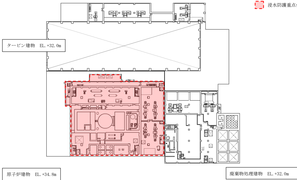
第 2.4-2 図(3) 浸水防護重点化範囲 (平面図)
