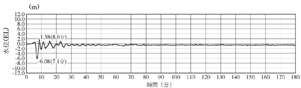
第2.5-1-3図 2号炉取水槽内の水位変動 (入力津波4, 防波堤無し, 循環水ポンプ運転時)
