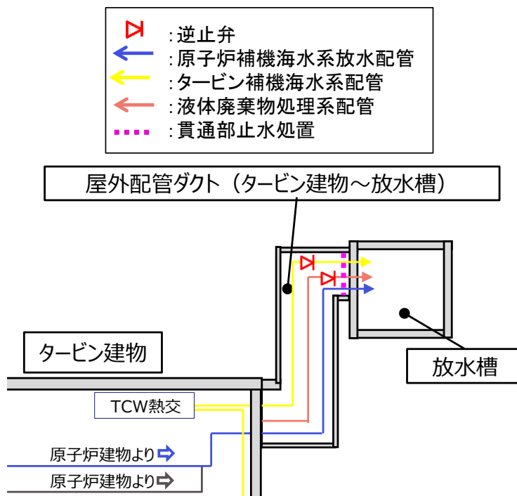
第 2.2-14-1 図 屋外配管ダクト平面図
