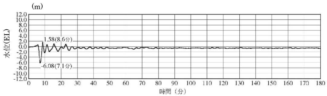
2号炉取水槽（入力津波4 防波堤無し）※下降側 ポンプ運転時
