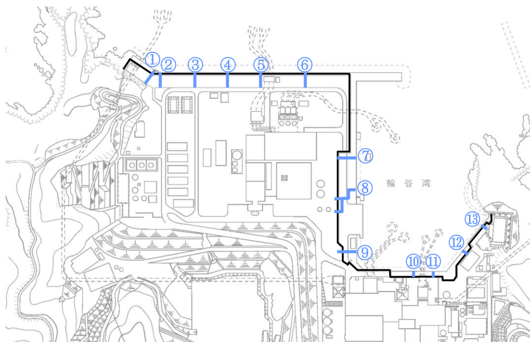
第2.2-15図 屋外排水路の全体配置図
