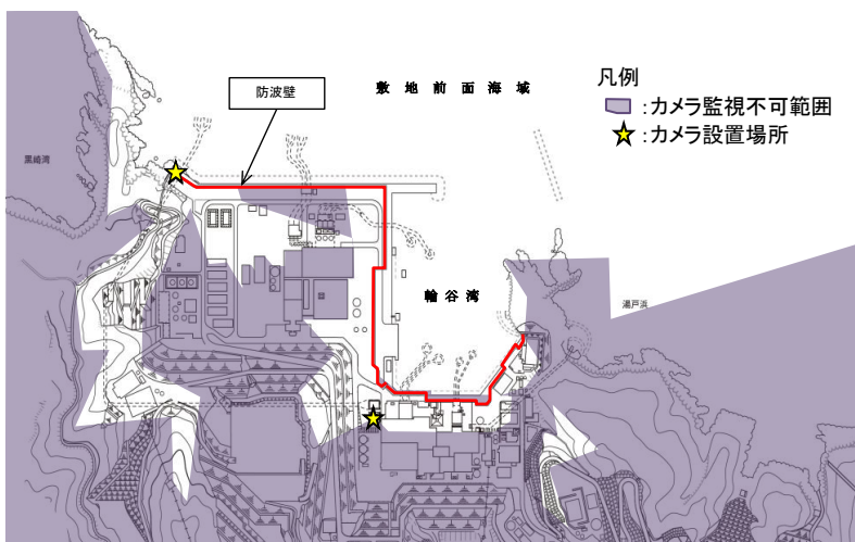
第4.3-5-2図 津波監視カメラが1台機能喪失した場合の視野範囲 (3号炉北側の防波壁上部東側E.L.+15.0m位置が機能喪失した場合)
