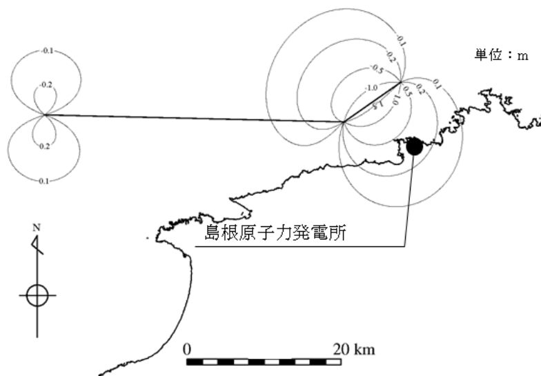
第 1.5-6 図 (5) (参考) 地殻変動量分布図：海域活断層上昇側最大ケース
