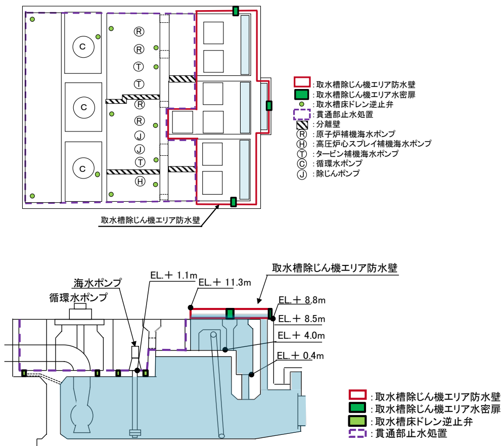
第4.2-4図 取水槽除じん機エリア防水壁配置図
