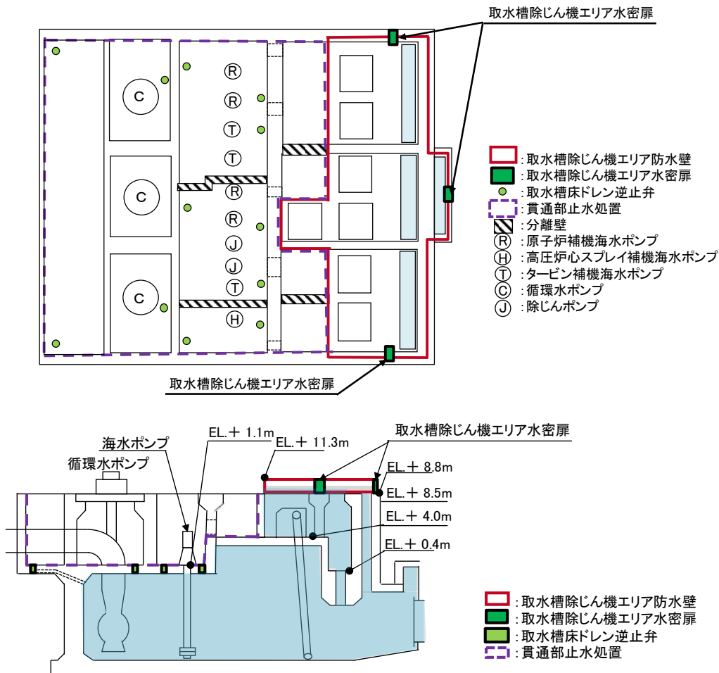
第4.2-7図 取水槽除じん機エリア水密扉配置図
