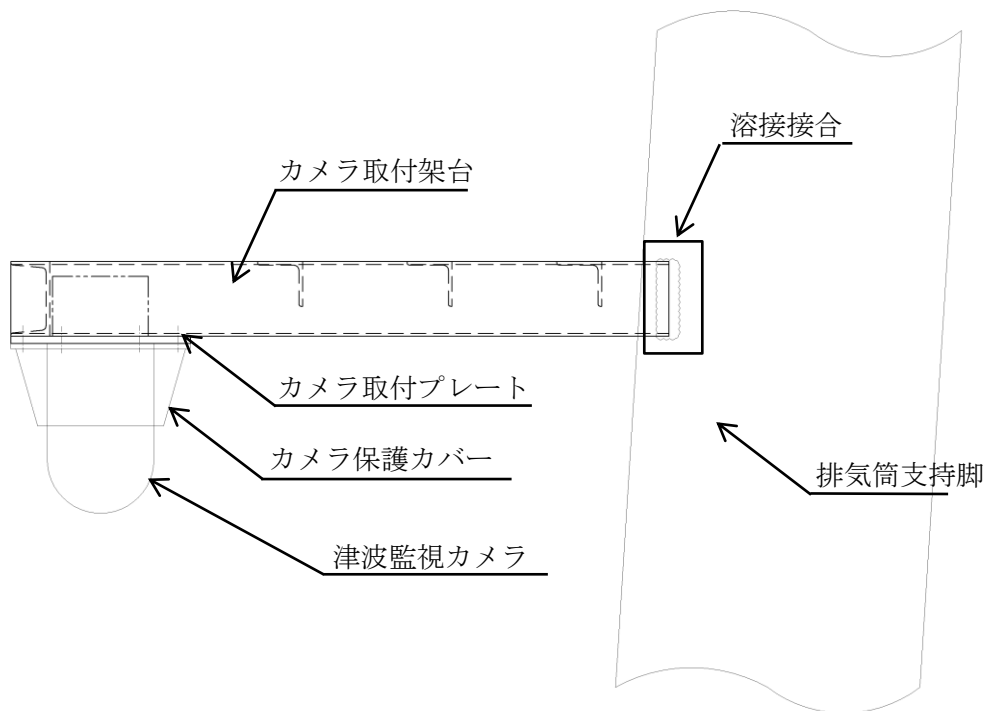
(断面図)
