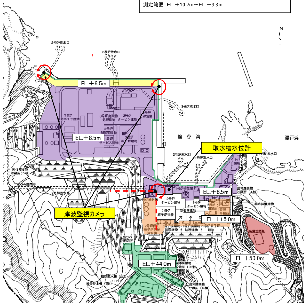
第4.3-1図 津波監視設備の配置
