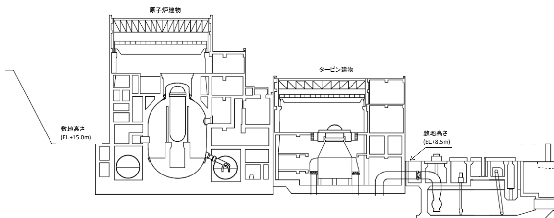
第 1.2-5 図 島根原子力発電所 2 号炉 主要断面図
