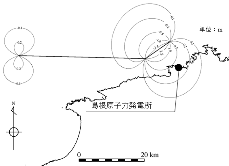
第 1.5-6 図 (4) 地殻変動量分布図：基準津波 4
