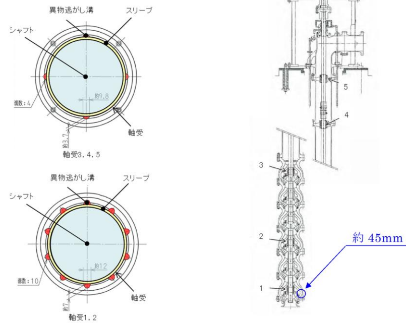
第3図 残留熱除去系海水系ポンプ 軸受部
