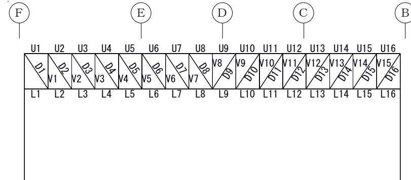
第 3-2 図 部材位置図
