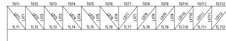
第 3-2 図 部材位置図 (主トラス)
