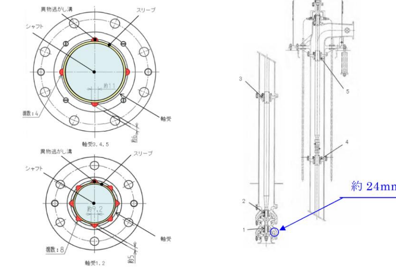
第5図 非常用ディーゼル発電機（高圧 炉心スプレイ系ディーゼル発電機を 含む。）用海水ポンプ軸受部
