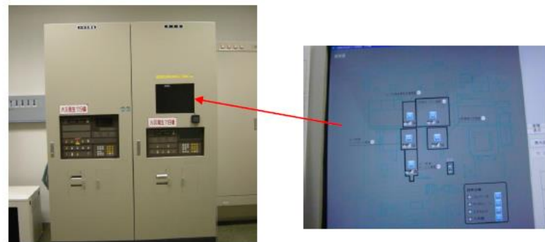
〈火災受信機盤・防災盤〉 〈地図式表示パネル〉
