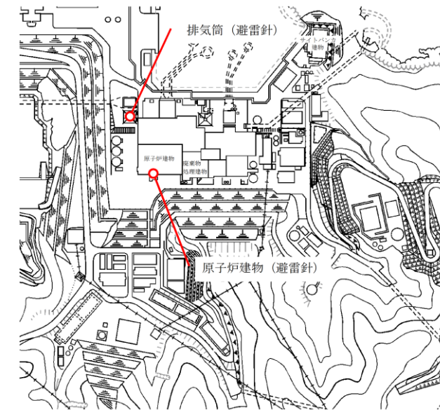
第 1-16 図 避雷設備の設置対象建物等
