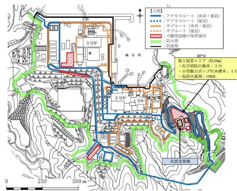
第 1-26図 移動式消火設備の配置の概要
