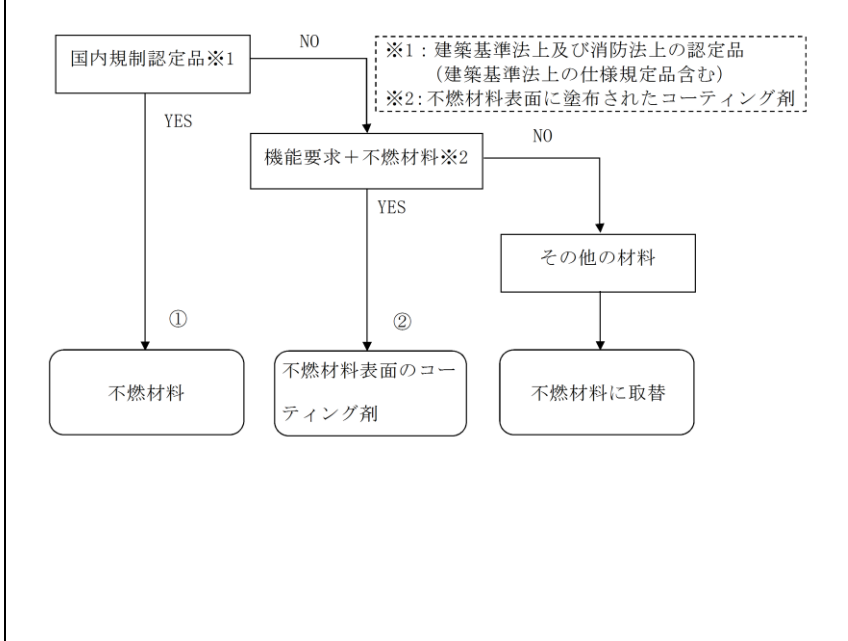
第1図 内装材の不燃性確認フロー
