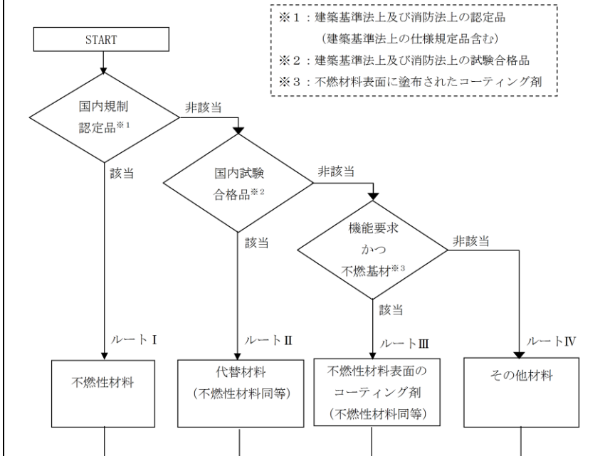
第1図 内装材の適合性判定フロー
