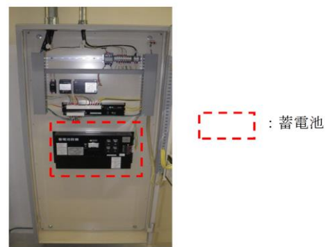
第1-31図 二酸化炭素自動消火設備（全域）制御盤内蓄電池
