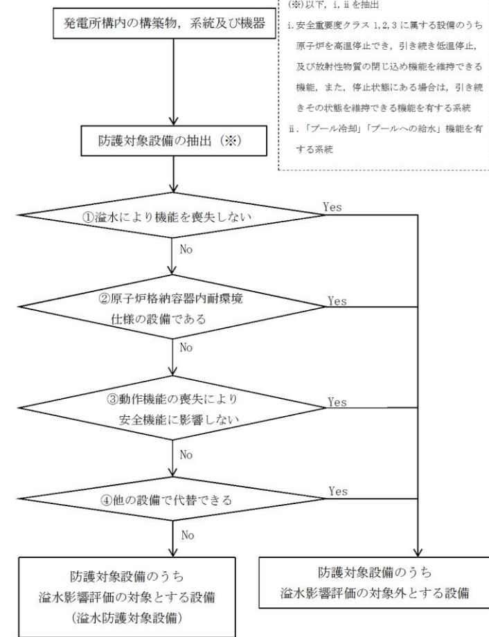
図2-1 防護対象設備のうち溢水影響評価の対象とする設備の選定フロー
