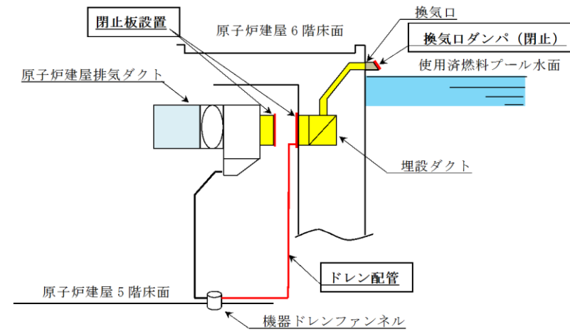
断面図
