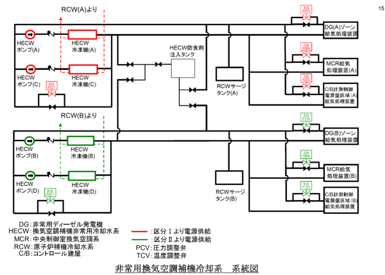
非常用換気空調補機冷却系系統図
