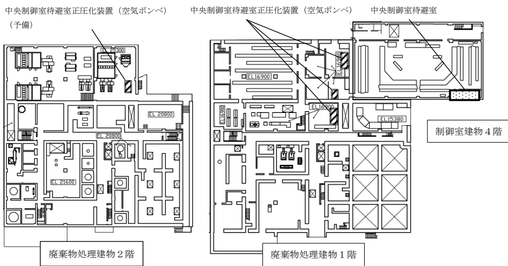
図 2.4-17 空気ボンベ設置 配置図
