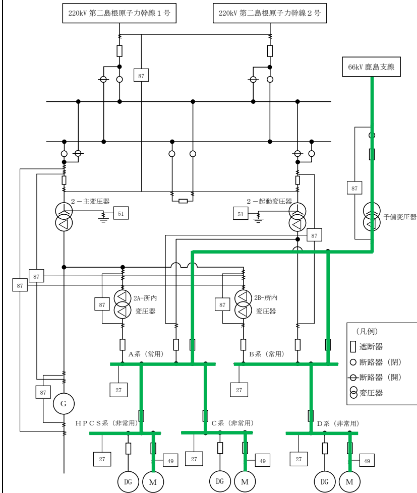
第7-1図 1相開放故障直前の状態
