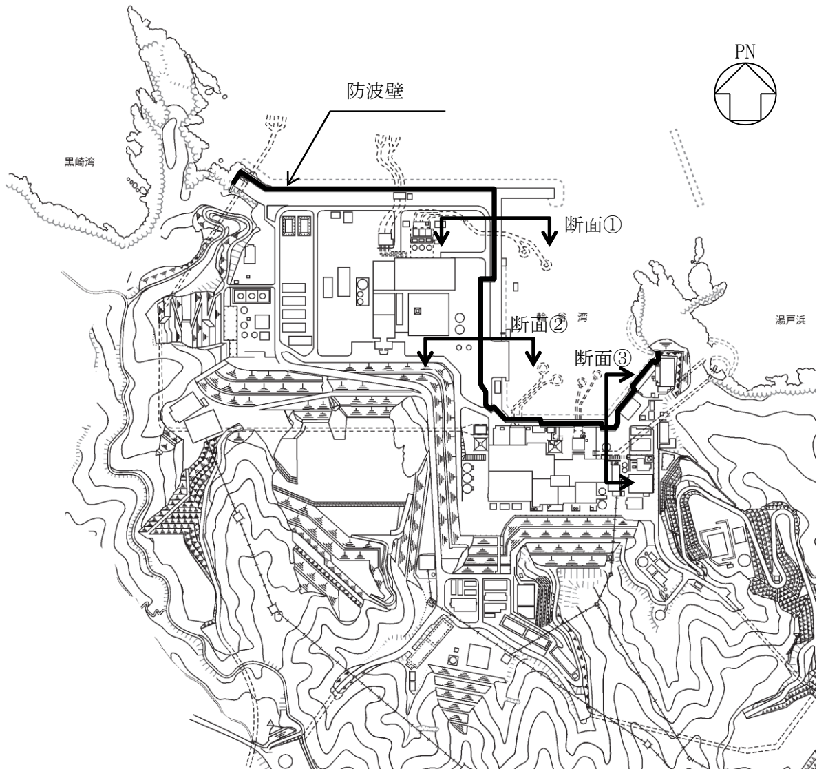
第 1 図 防波壁配置図
