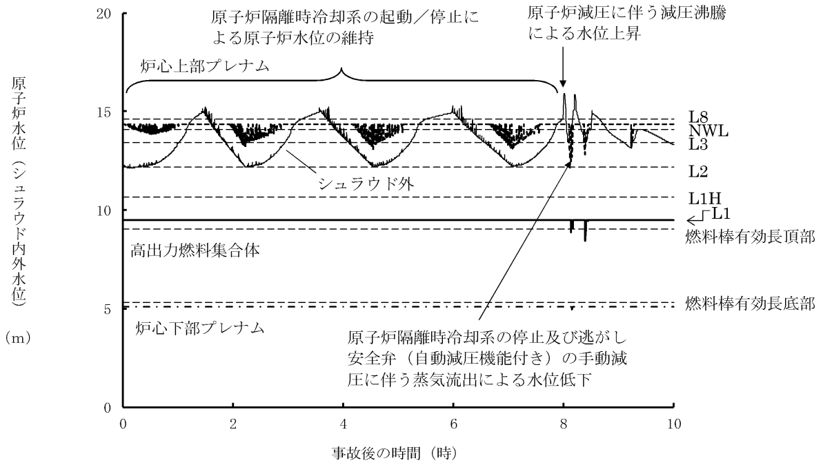
第 2.4.1.2-1(3) 図 原子炉水位（シユラウド内外水位）の推移
