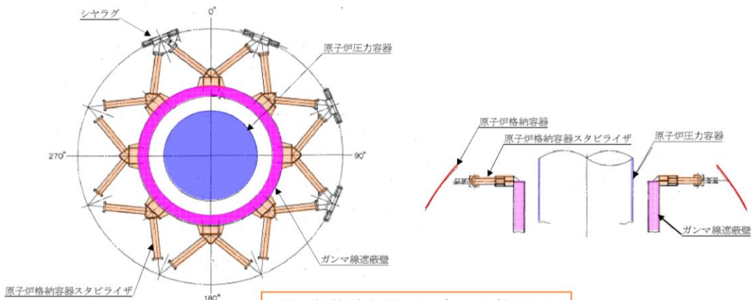
原子炉格納容器スタビライザ概要図
