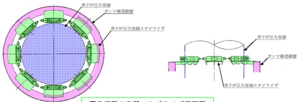
原子炉圧力容器スタビライザ概要図
