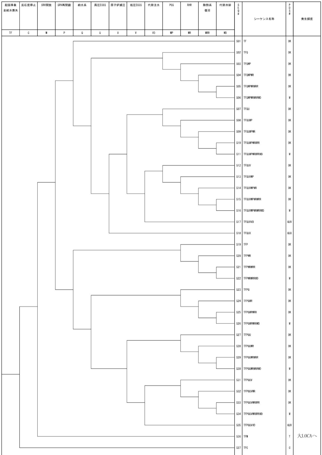
第6図 全給水喪失に対するイベントツリー
