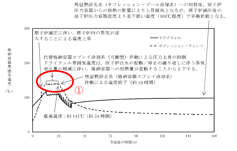
第 2.3.2-14 図 格納容器雰囲気温度の推移
