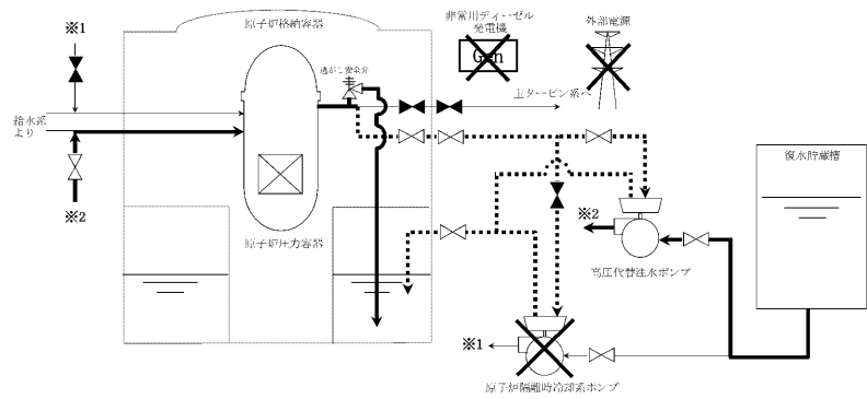
第 2.3.2.1 図 「全交流動力電源喪失 (外部電源喪失+DG 喪失)+RCIC 失敗」の重大事故等対策の概略系統図 (1/4) (原子炉注水)
