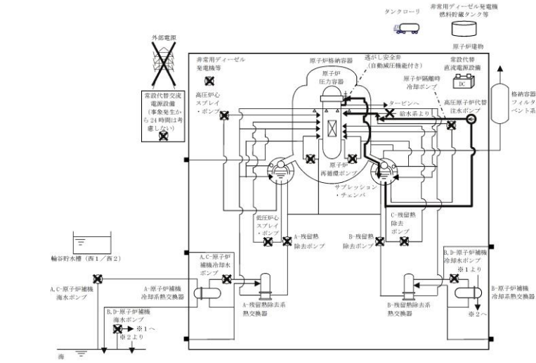
第 2.3.2.1-1(1) 図 「全交流動力電源喪失 (TBU)」の重大事故等対策の概略系統図 (原子炉注水)
