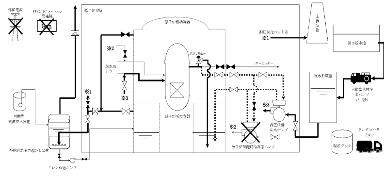
第 2.3.2.2 図 「全交流動力電源喪失 (外部電源喪失+DG 喪失)+RCIC 失敗」の重大事故等対策の概略系統図 (2/4) (原子炉注水及び原子炉格納容器除熱)
