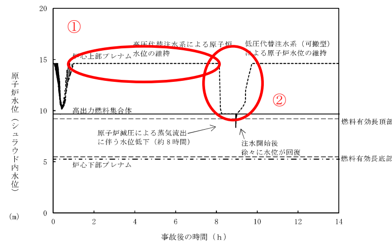
第 2.3.2-5 図 原子炉水位 (シユラウド内水位) の推移
