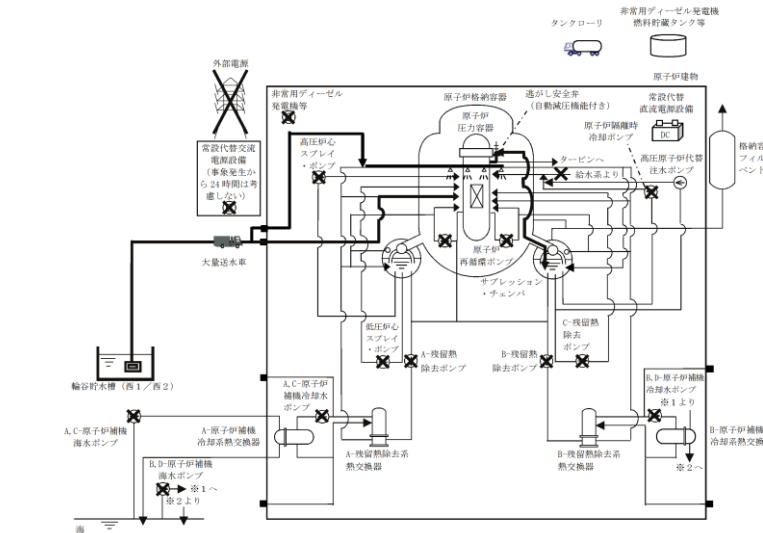
第 2.3.2.1-1(2) 図 「全交流動力電源喪失 (TBU)」の重大事故等対策の概略系統図 (原子炉減圧, 原子炉注水及び原子炉格納容器冷却)
