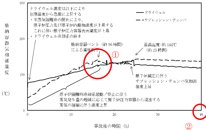
第 2.3.1.17 図 格納容器気相部温度の推移
