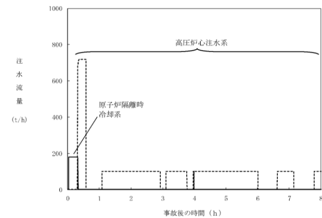
第 2.7.9 図 注水流量の推移
