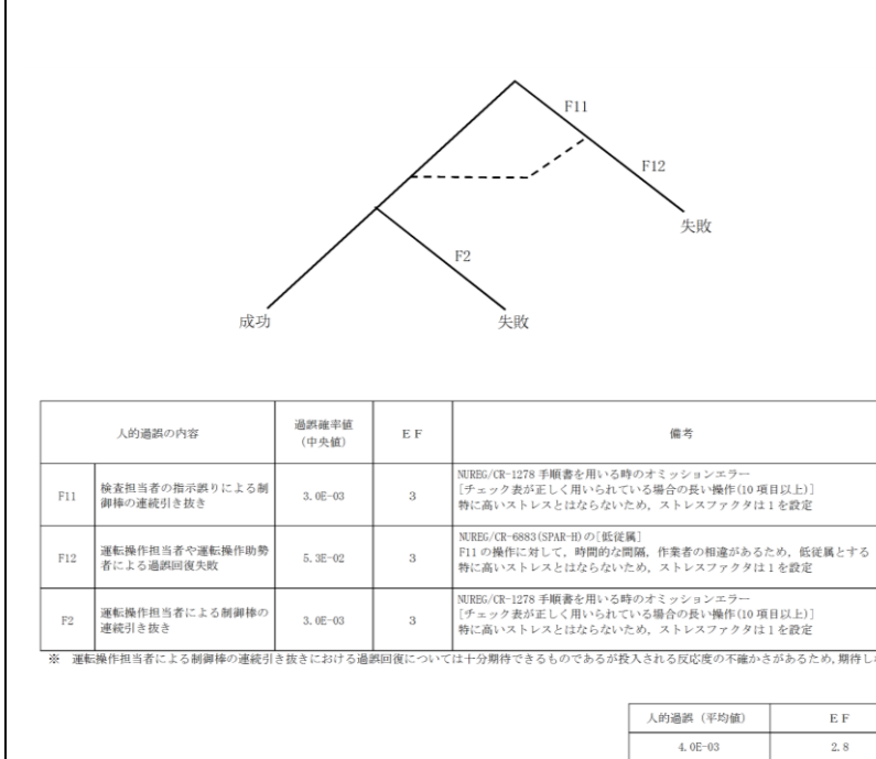
図1 「c. 制御棒の連続引き抜き」のHRA ツリー及び人的過誤確率
