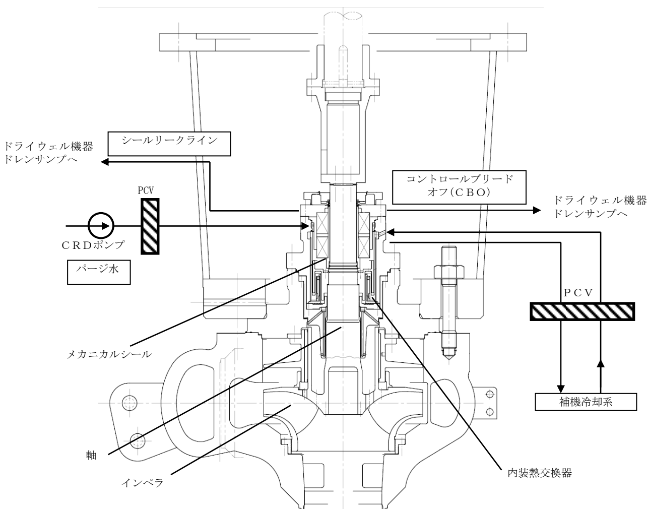
図1 PLRポンプ 概略図
