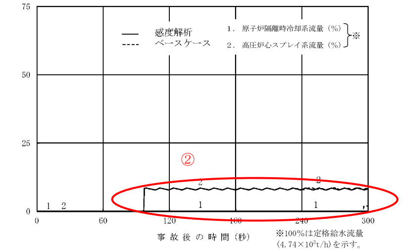
図3 原子炉隔離時冷却系, 高圧炉心スプレイ系の流量の推移 (事象発生から 300 秒後まで)
