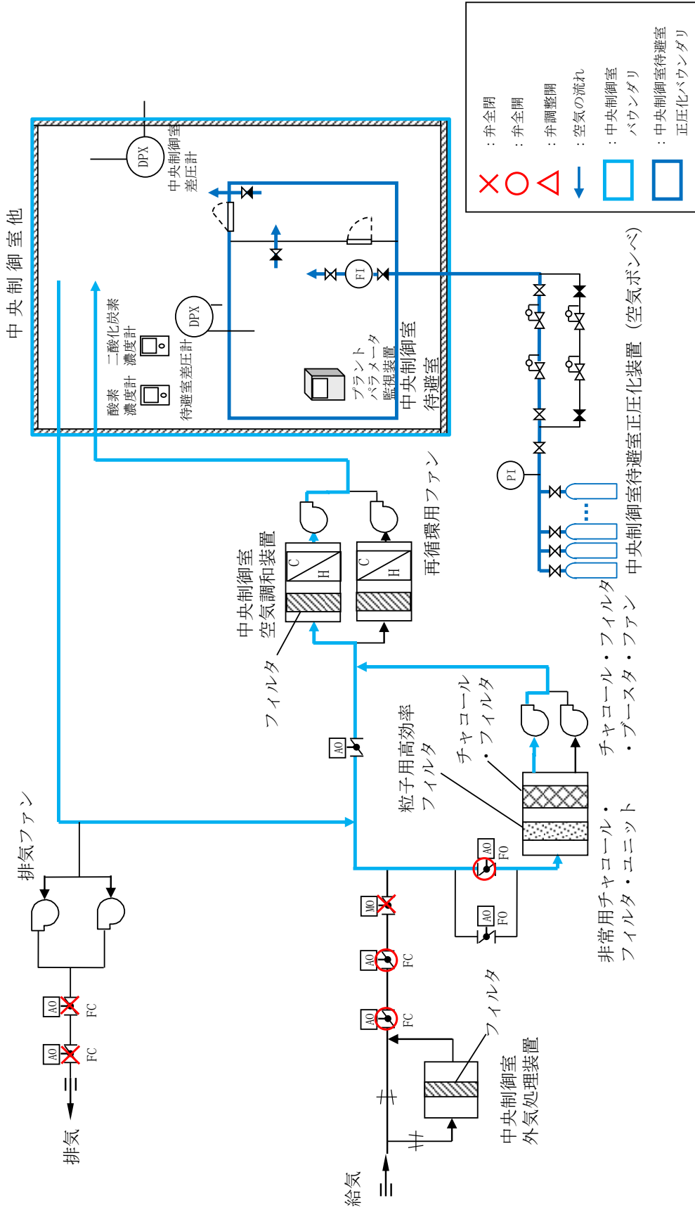
図 3 (2 / 2) 中央制御室換気系及び中央制御室待避室正圧化装置 (空気ボンベ) 概略系統図 (非常時運転モード (加圧運転 (プルーム通過中)))
