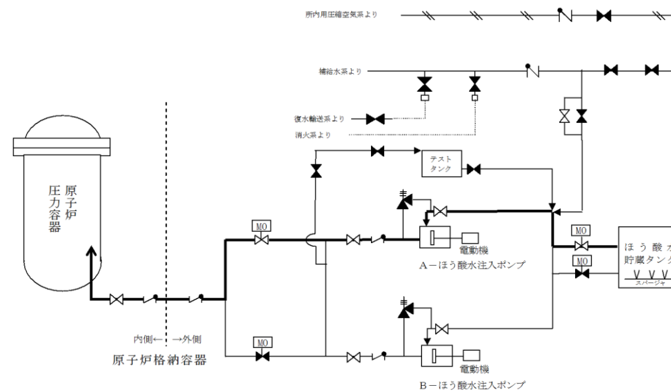
図6 ほう酸水注入系 設備概要
