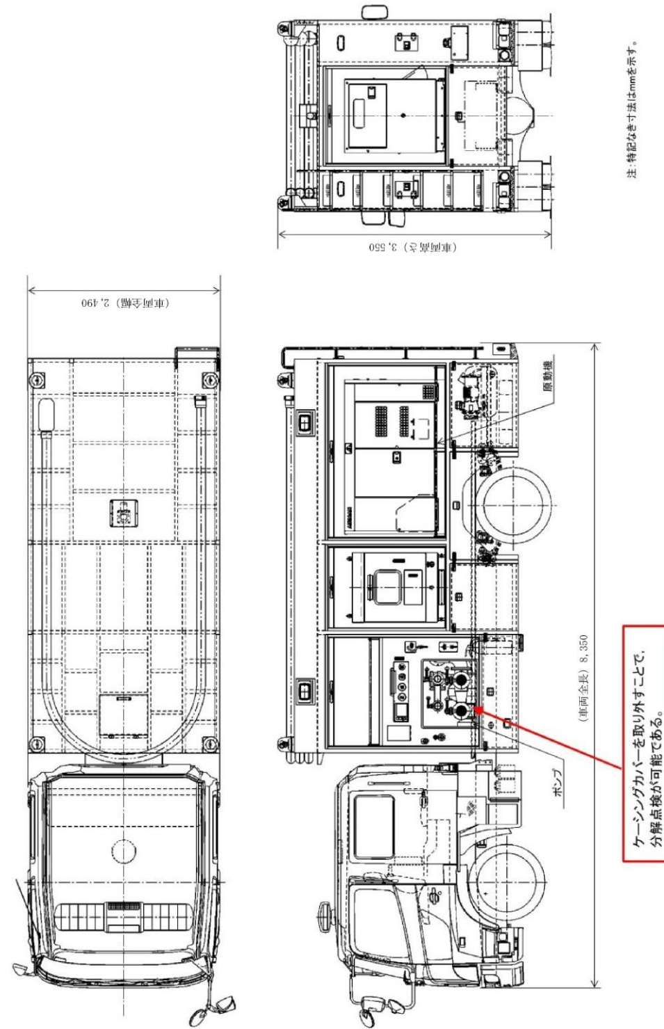
図6 構造図 (大量送水車)
