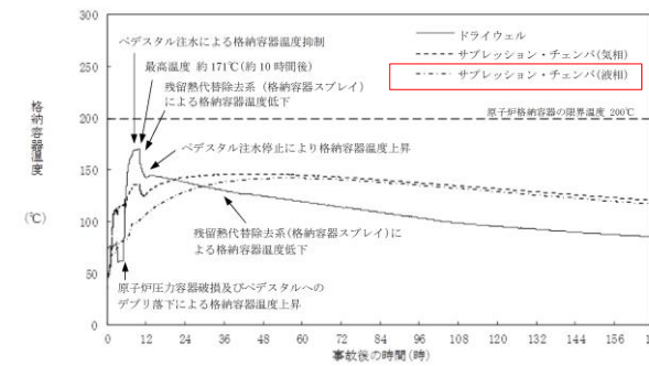
図2 サプレッション・チェンバ・プール水温の推移 (格納容器スプレイ及び格納容器スプレイによる原子炉格納容器下部への注水)
