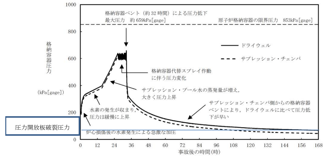
図 13 原子炉格納容器圧力推移 (冷却材喪失 (大破断 LOCA) + ECCS 注水機能喪失 + 全交流動力電源喪失)
