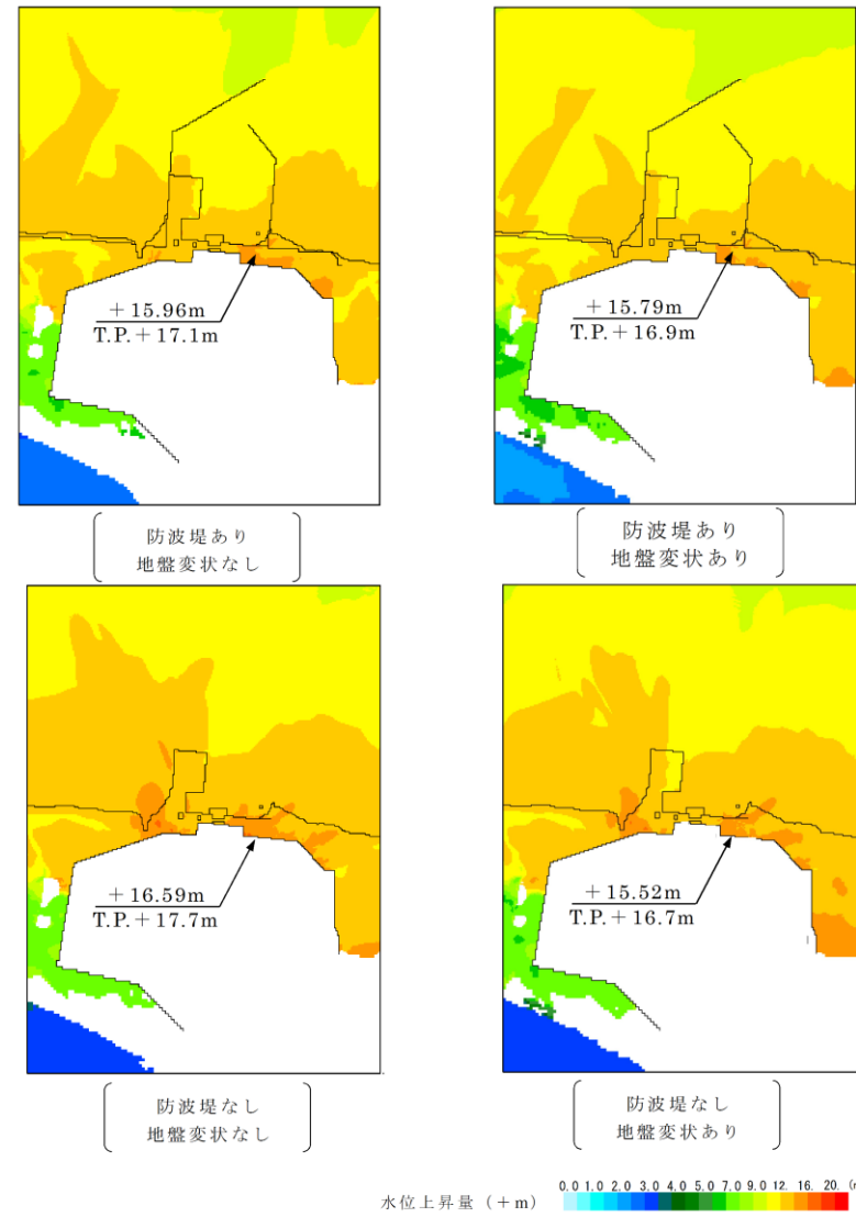
第 2. 1. 3-1 図 基準津波による最大水位上昇量分布 防潮堤ルート変更前を示す。
