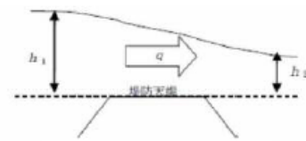
図 4 本間公式
