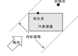
図10 風向に垂直な建屋投影面積の考え方
