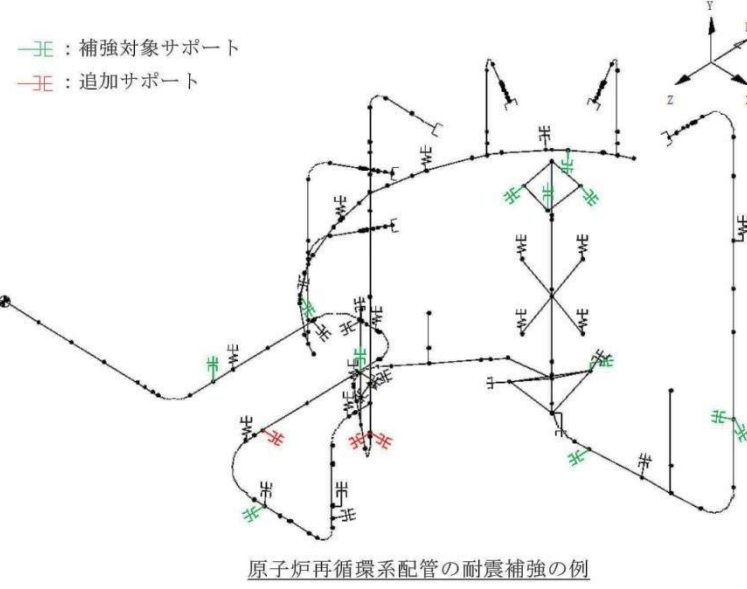
第5図 配管系の耐震補強概要図
