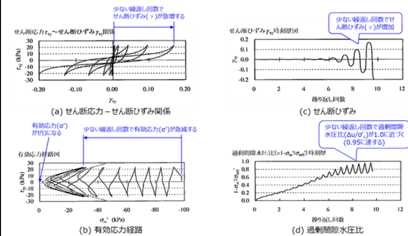
第3-2-5 図 緩い砂の液状化試験結果
