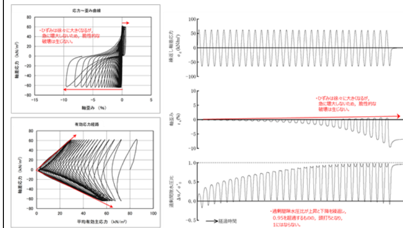
第3-2-14 図 液状化試験結果の例 (A地点の埋戻土 (掘削ズリ))
