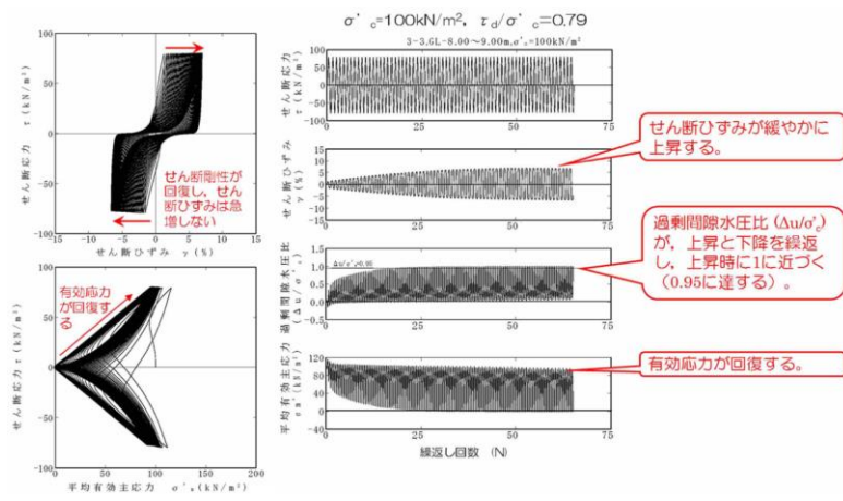
第11-4-9 図 液状化試験結果の例 (A-1 地点の洪積砂層 I)
