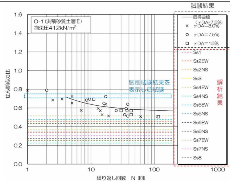
第11-6-11 図 累積損傷度理論に基づく評価結果 (0-1 地点の洪積砂質土層Ⅱ)
