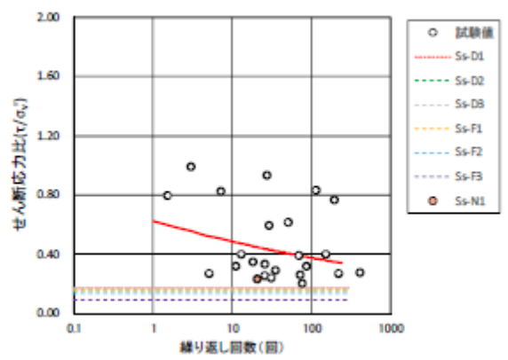
(a) 盛土
