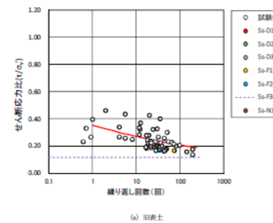
(a) 旧表土
