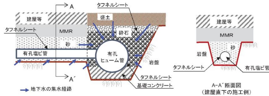
添付 1-9 図 有孔塩ビ管と有孔ヒューム管の接続概念
