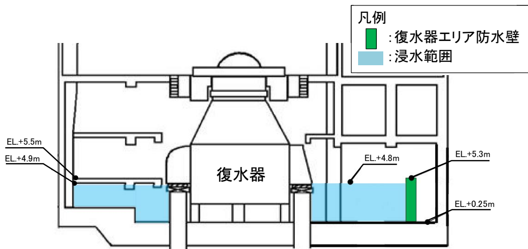
(A-A 断面)
