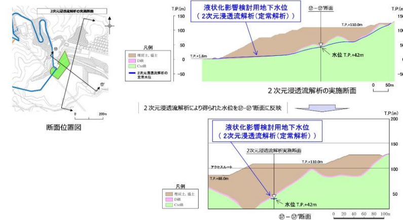
第 4.4-4 図 2次元浸透流解析による検討用地下水位 (上図：2次元浸透流解析の実施断面，下図：①-①'断面)
