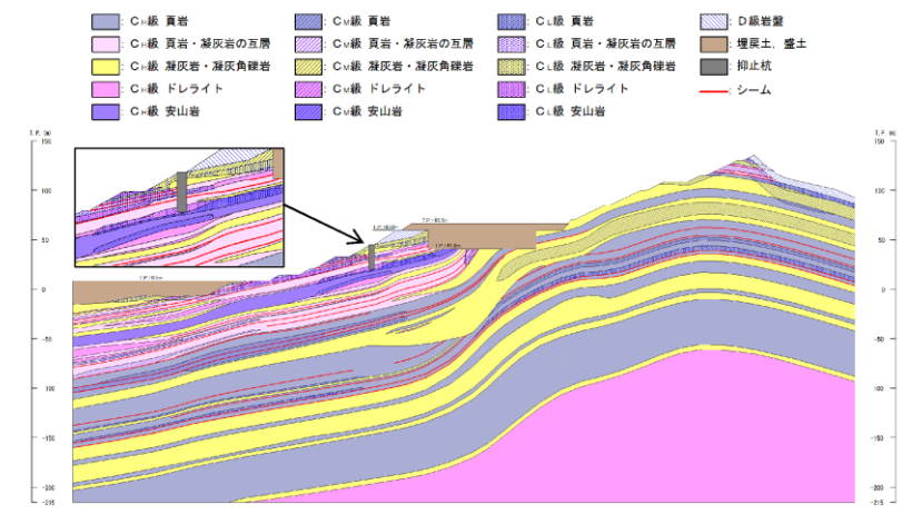
第 7. 4. 3-4(1) 図 ②-②' 断面 解析用岩盤分類図
