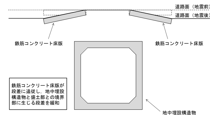
第2図 段差緩和対策例 (沈下後)
