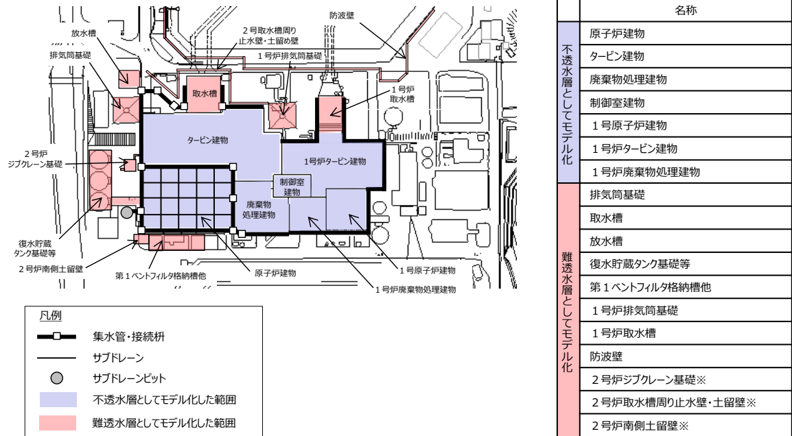
別紙17-7図 主要建物周辺における構造物等のモデル化方針
