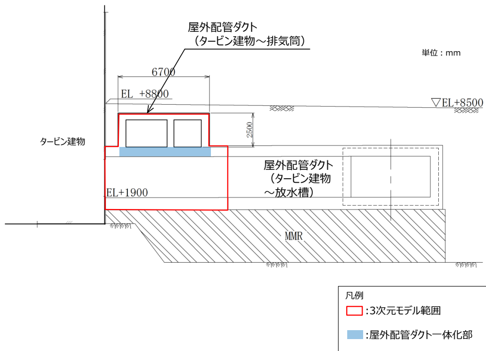
第6-2-63図 屋外配管ダクト (タービン建物～排気筒) 断面図 (②-②断面)
