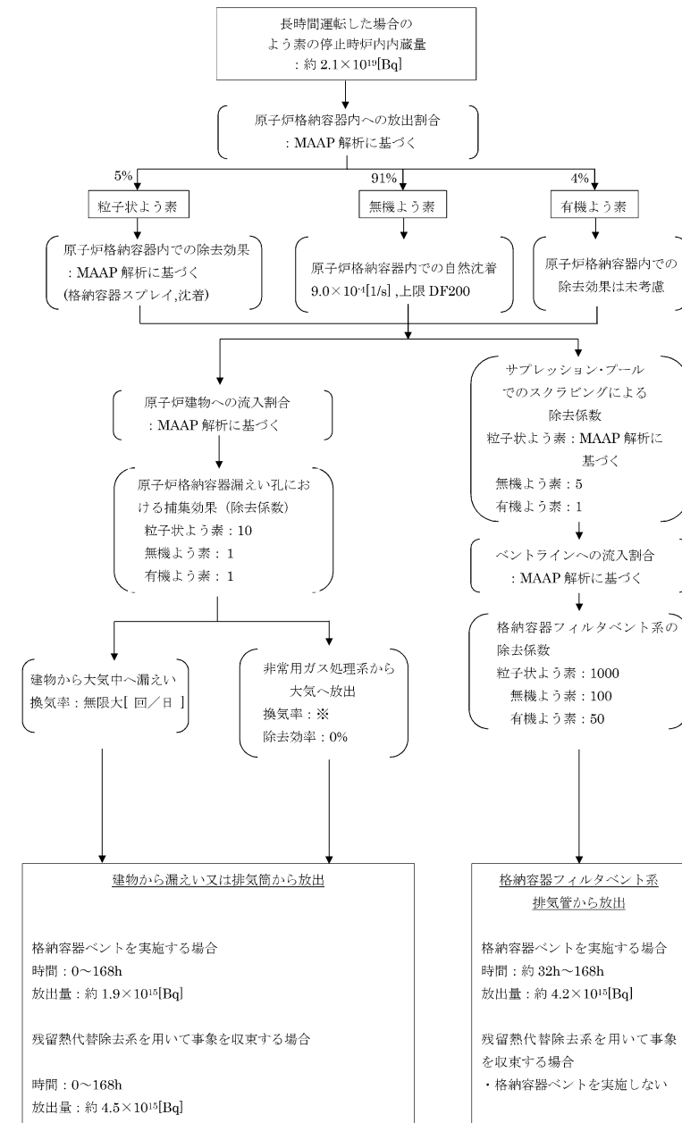
図2 よう素の大気放出過程
