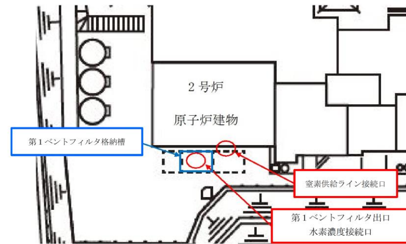
第10図 屋外作業場所
