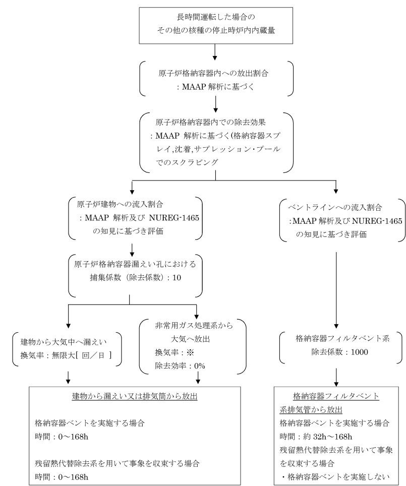
図4 其他核種の大気放出過程
