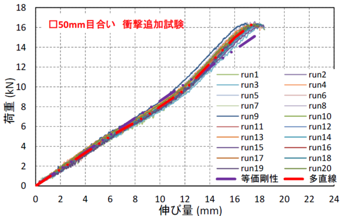
第2-1図 ネットの交点引張試験結果
