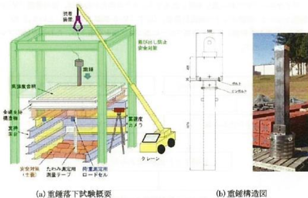
第 2-1 図 試験概要図
