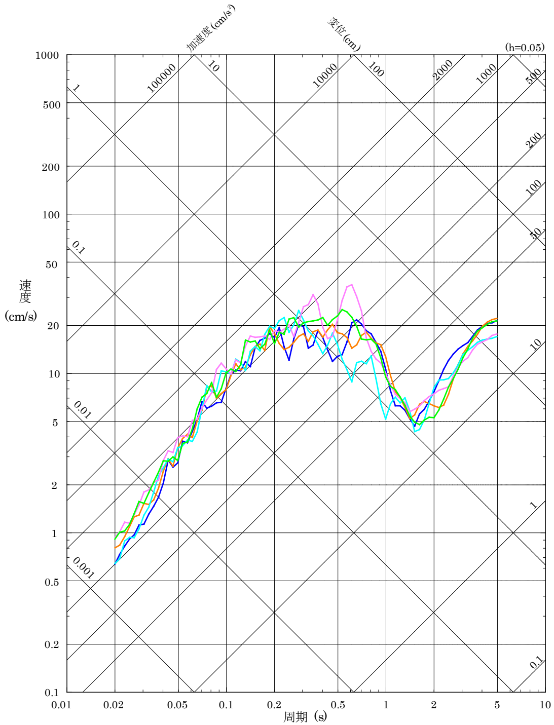
第 5.6-11 図 (12) 「F-Ⅲ断層 + F-Ⅳ断層 + F-Ⅴ断層による地震」の断層モデルを用いた手法による地震動評価結果 (鉛直方向) (アスペリティの不確かさを考慮したケース (一塊: 縦長))
