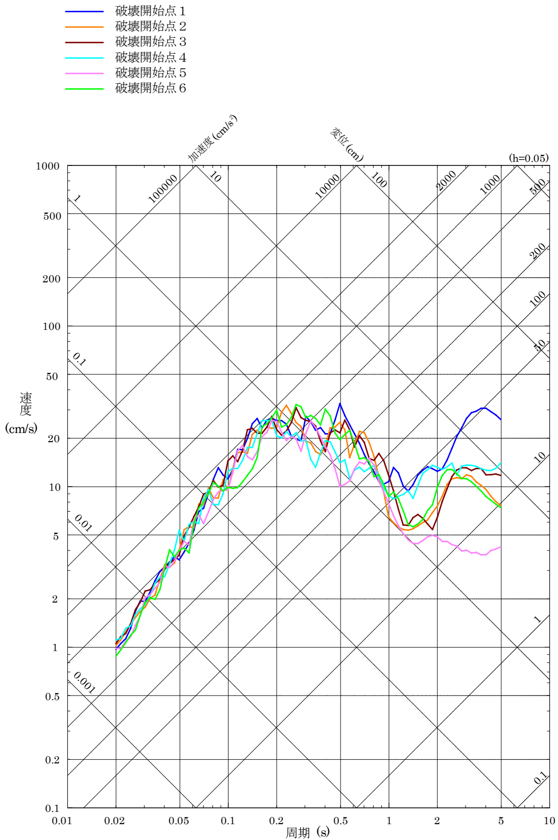
第 5.6-11 図 (14) 「F-Ⅲ断層 + F-Ⅳ断層 + F-V断層による地震」の断層モデルを用いた手法による地震動評価結果 (鉛直方向) (中越沖地震の短周期レベルの不確かさを考慮したケース)
