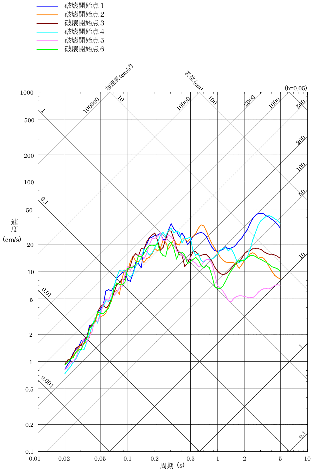
第 5.6-11 図 (6) 「F-Ⅲ断層 + F-Ⅳ断層 + F-V断層による地震」の断層モデルを用いた手法による地震動評価結果 (鉛直方向) (破壊伝播速度の不確かさを考慮したケース)
