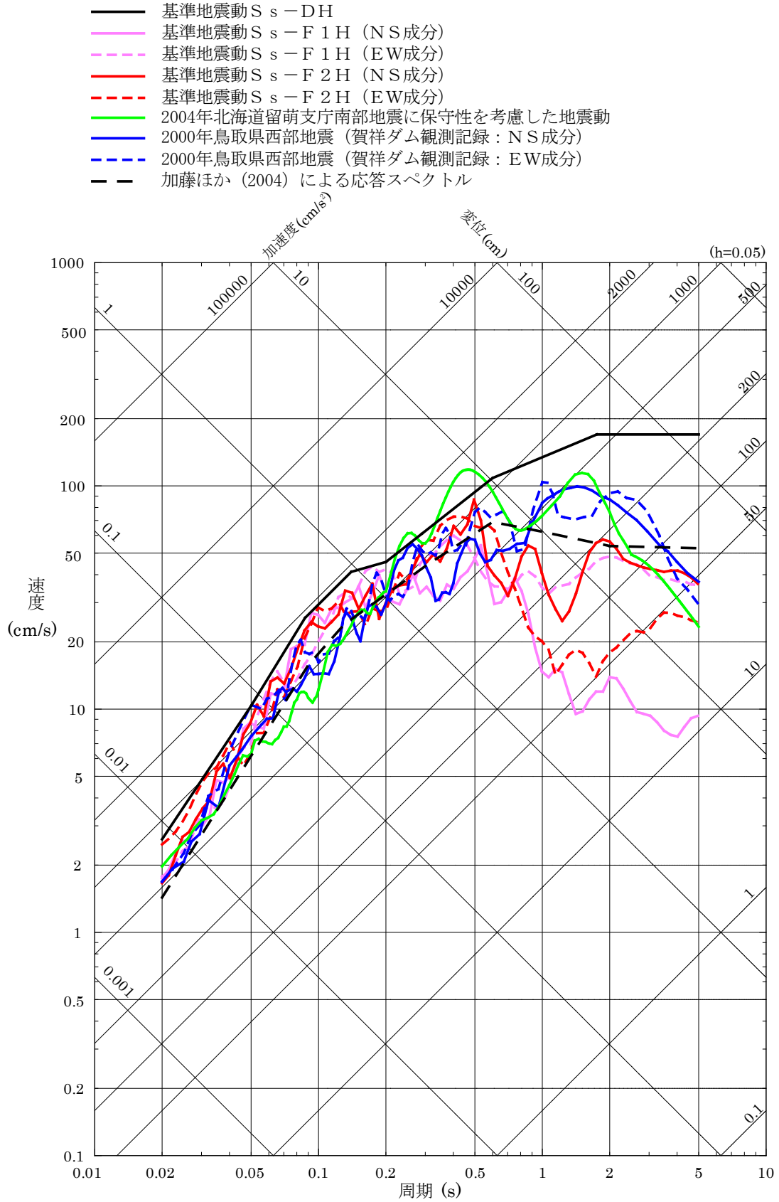
第 5.6-18 図(1) 震源を特定せず策定する地震動と敷地ごとに震源を特定する地震動による基準地震動 S_s の応答スペクトル (水平方向)
