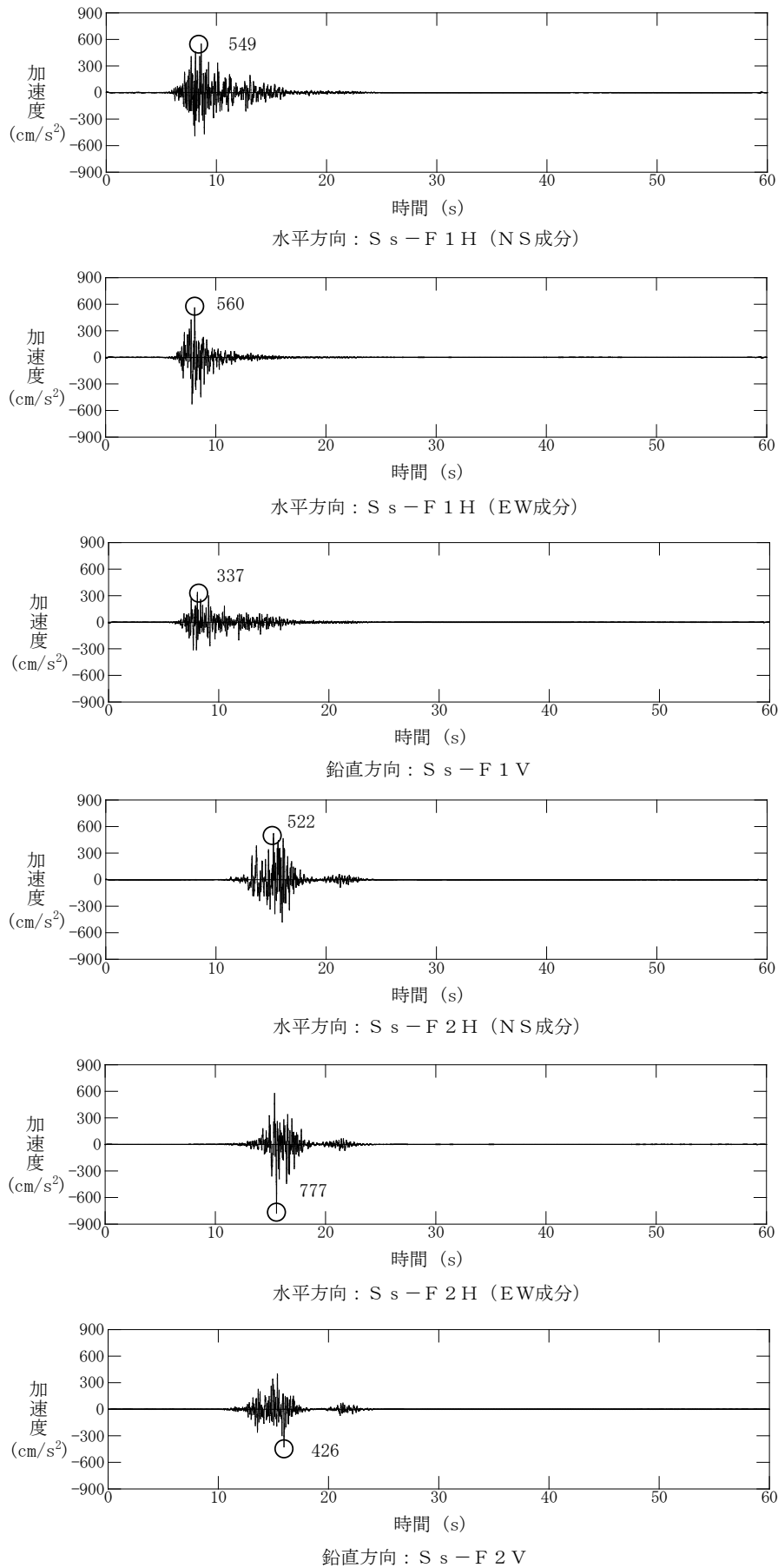
第 5.6-21 図 基準地震動 S s - F 1 及び S s - F 2 の時刻歴波形
