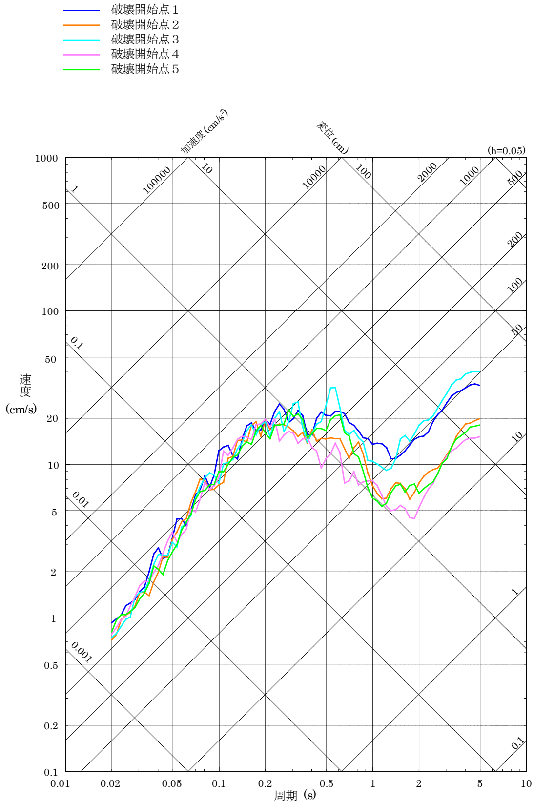
第 5.6-11 図 (10) 「F-Ⅲ断層 + F-Ⅳ断層 + F-Ⅴ断層による地震」の断層モデルを用いた手法による地震動評価結果 (鉛直方向) (アスペリティの不確かさを考慮したケース (一塊: 横長))
