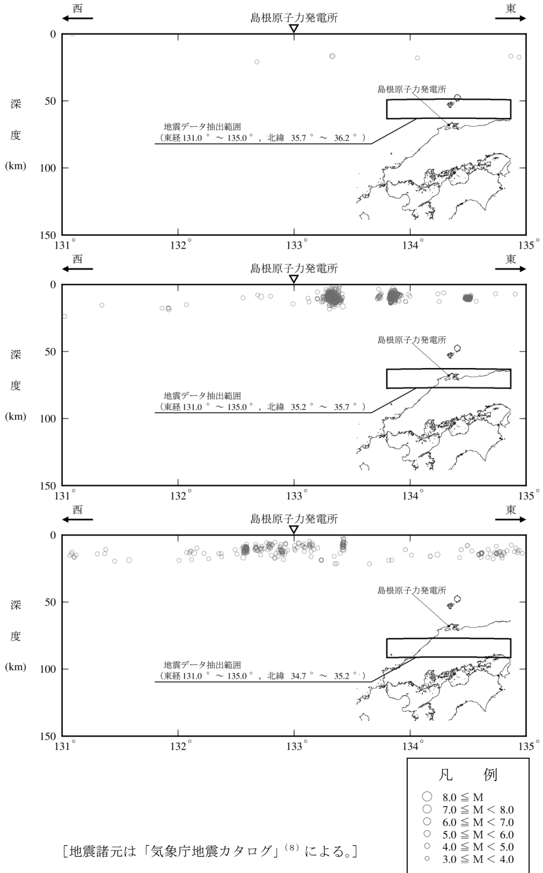
第 5.2-4 図 (2) 敷地周辺における地震 (M ≥ 3) の震源鉛直分布 (東西方向) (1997 年 10 月 ~ 2019 年 8 月)
