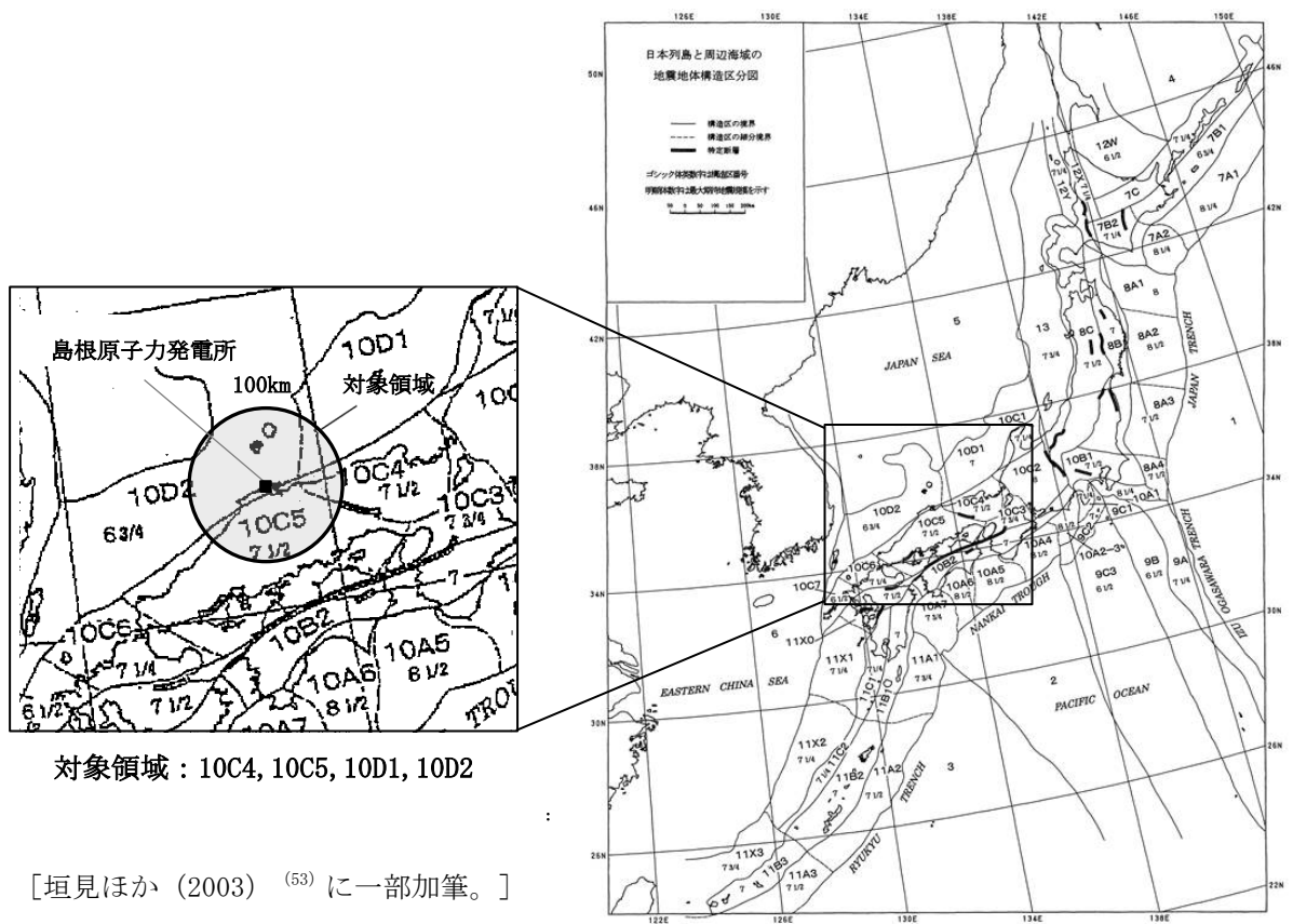
(b) 垣見ほか(2003) (53) に基づく対象領域
