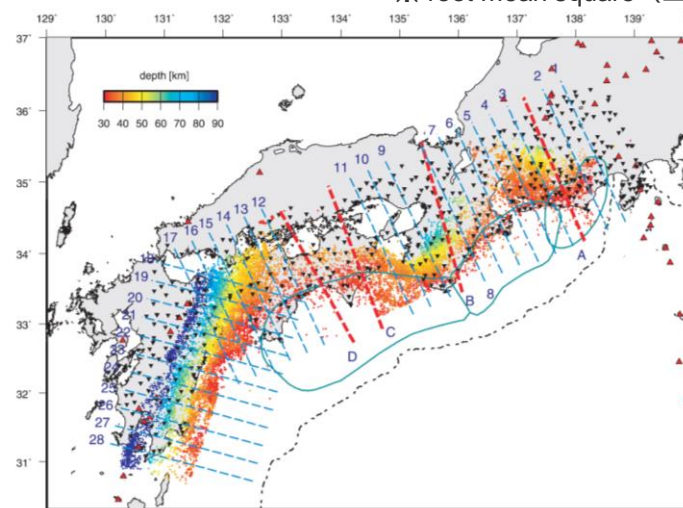
<解析対象地震> (弘瀬・他(2007)による)
