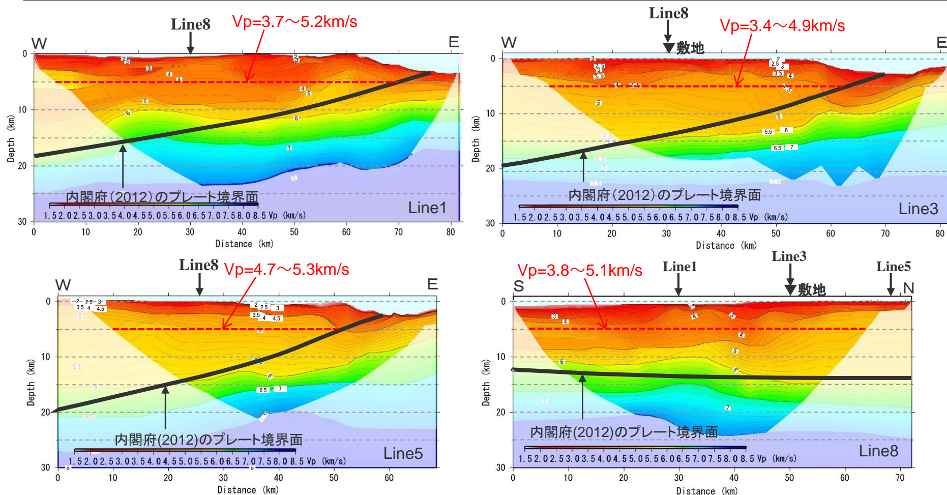
<屈折法地震探査によるP波速度構造 (Line1,3,5,8) >
