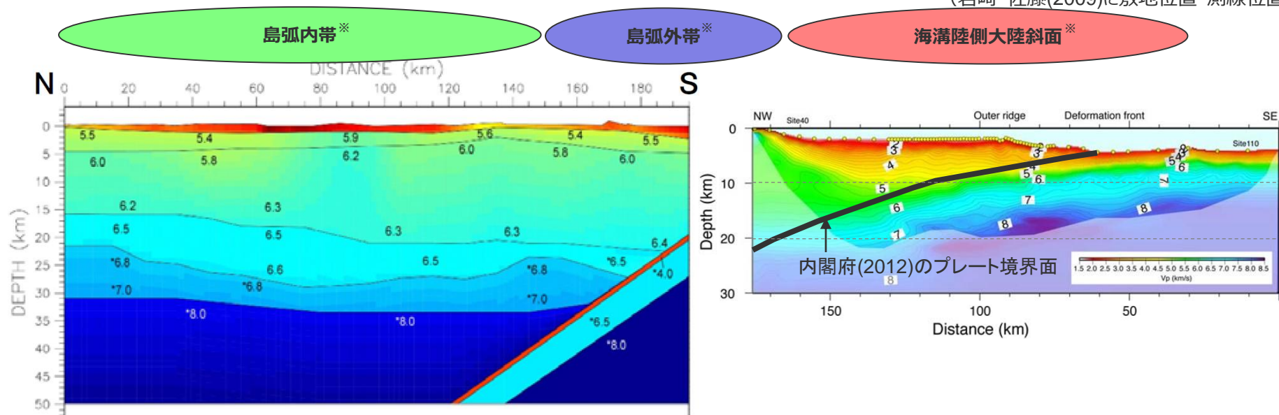
<近畿地方のP波速度構造 (廣瀬・伊藤(2006)及びNakanishi et al.(2008)に地震地体構造区分・プレート境界面を重ね描き) >
