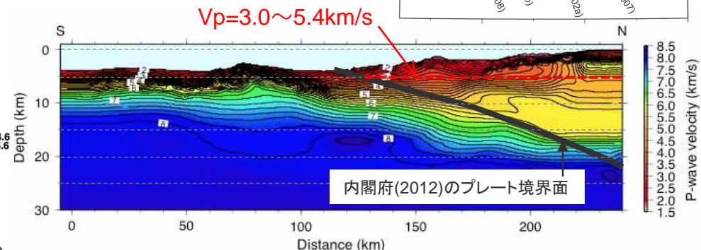
(東京大学地震研究所(2007)にプレート境界面を重ね描き、深さ5kmのVpを加筆)
