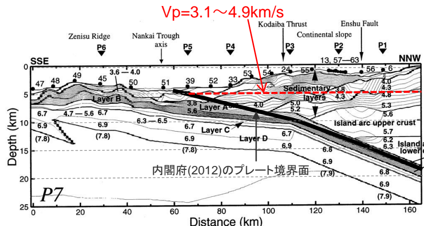
(Nakanishi et al.(2002a)にプレート境界面を重ね描き、深さ5kmのVpを加筆)
