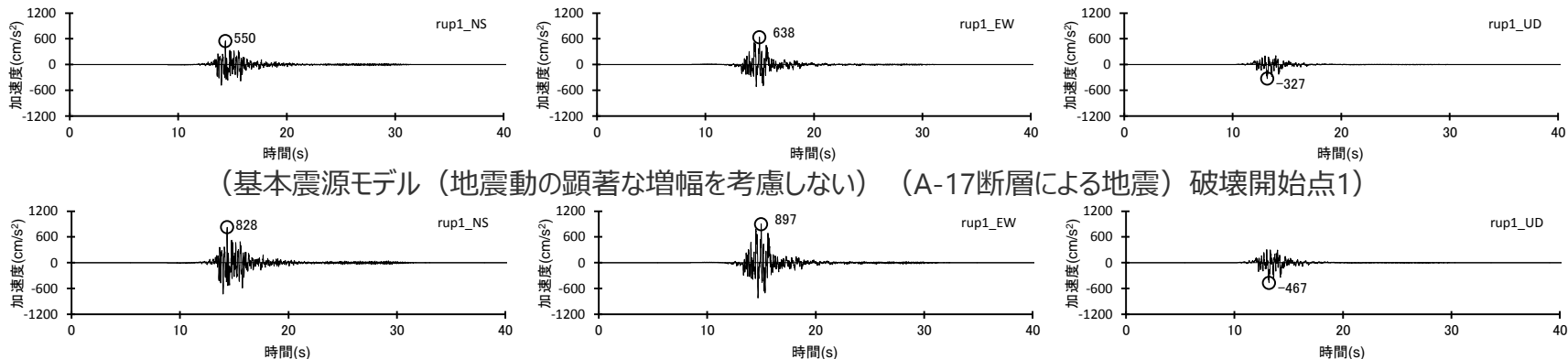
(アスペリティの応力降下量の不確かさを考慮した震源モデル（地震動の顕著な増幅を考慮しない） (A-17断層による地震) 破壊開始点1)
