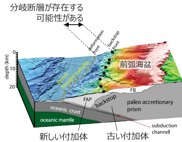
分岐断層が存在する可能性がある 新しい付加体 古い付加体 <チリの分岐断層の地形> (Contreras-Reyes et al.(2010)に図の説明 (前弧海盆、新しい付加体、古い付加体)、分岐断層が存在する可能性がある旨を加筆)
