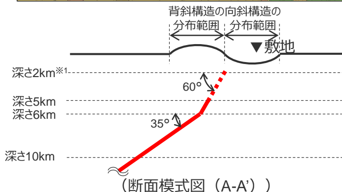
＜A-17断層による地震の断層面※1,2＞
