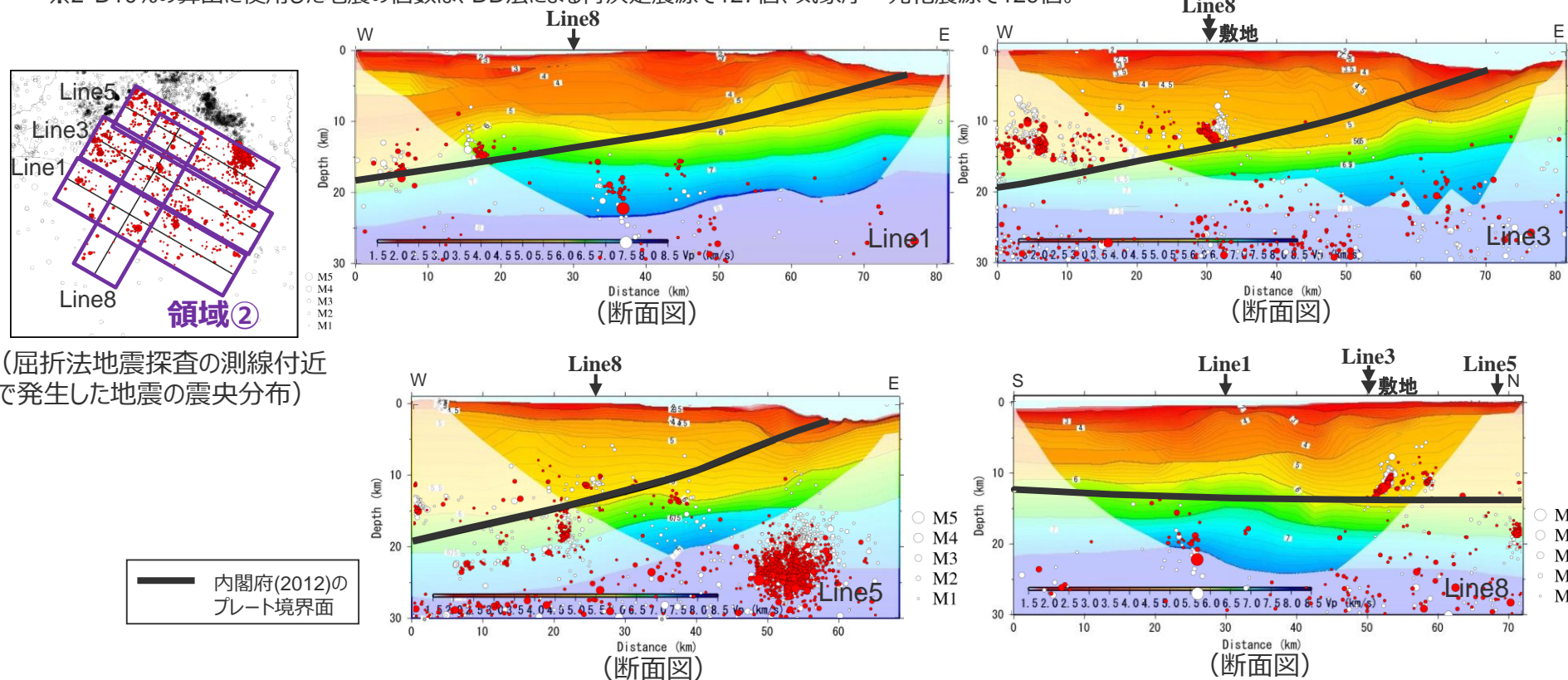
<屈折法地震探査によるP波速度構造 (Line1,3,5,8) と震源鉛直分布> (観測分析期間: 1997年10月~2015年12月)
