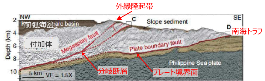
<南海トラフを切る反射断面（左図B断面）>
