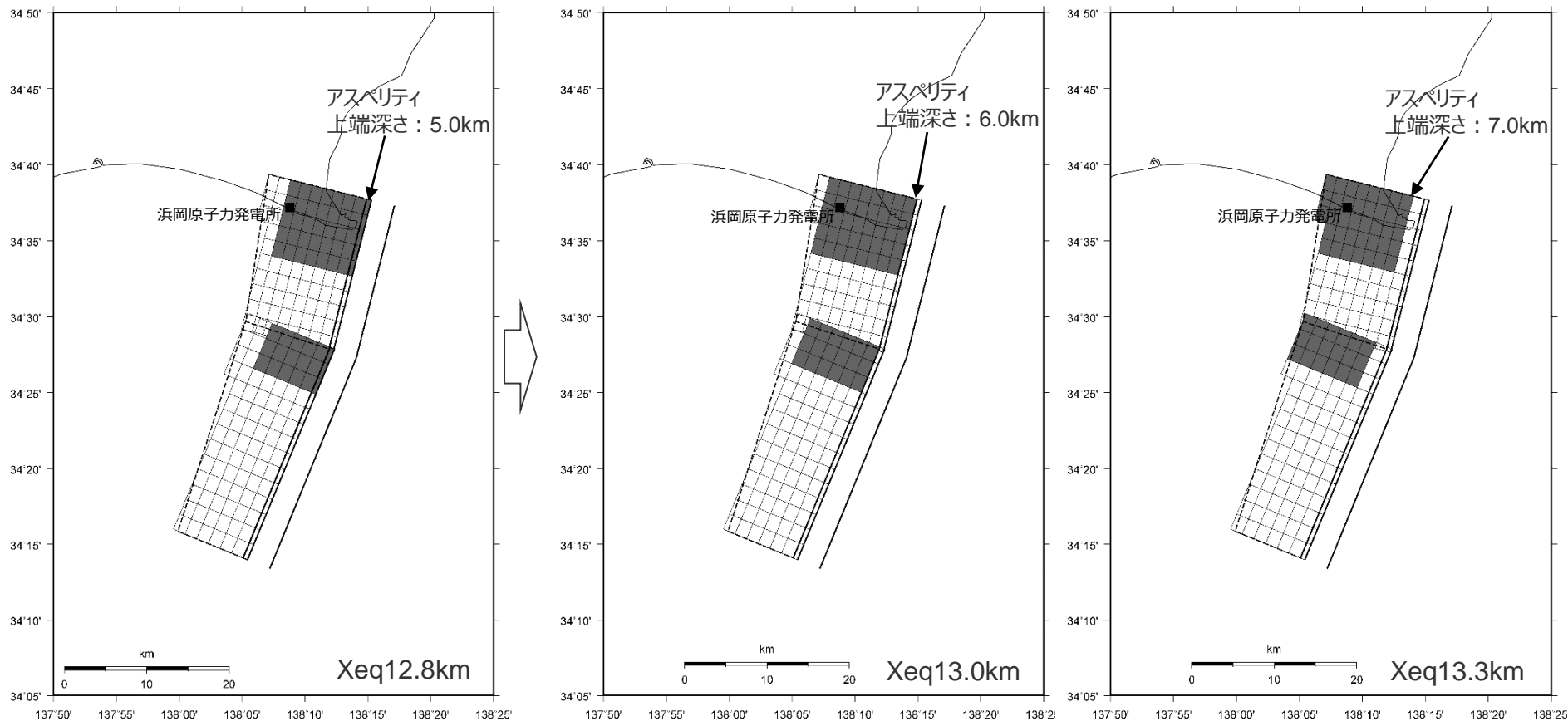
<基本震源モデル（地震動の顕著な増幅を考慮しない）>
