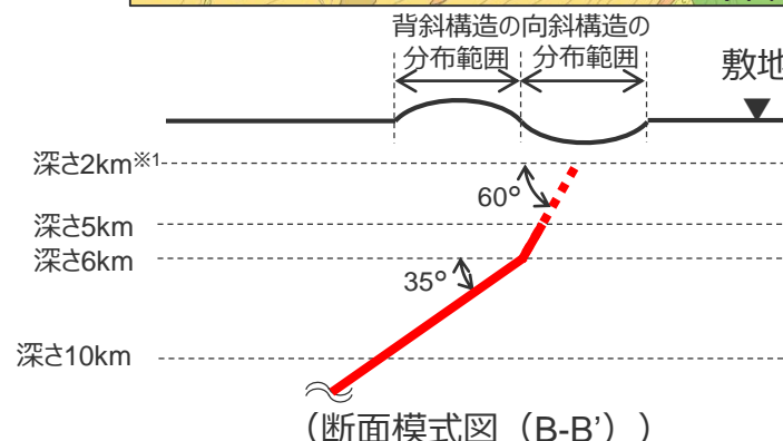
＜A-5・A-18断層による地震の断層面※1＞
