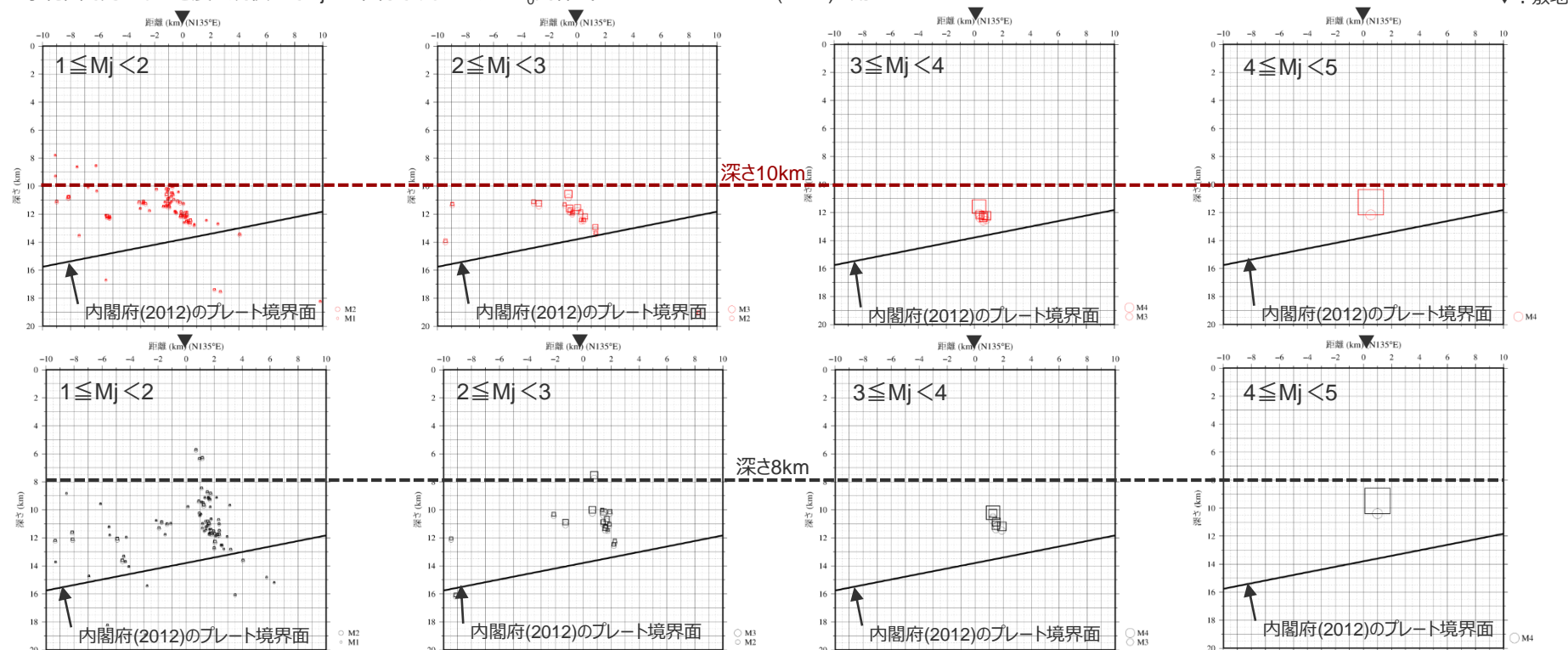
<敷地を中心に20km四方 (±10km) の範囲におけるDD法による再決定震源及び気象庁一元化震源に基づく想定震源断層面の鉛直分布 (観測分析期間: 1997年10月~2015年12月、深さ20km以浅) >
