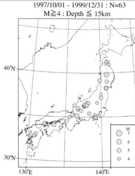
<M4以上の内陸の浅い自然地震分布 (S波速度構造算定用)>
