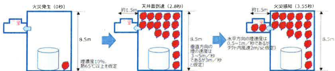
第 3-6-5-5-3 図 化学体積制御設備脱塩塔バルブ室及び使用済燃料ピット脱塩塔バルブ室のうち脱塩塔室内での火災発生時の空気の流れ
