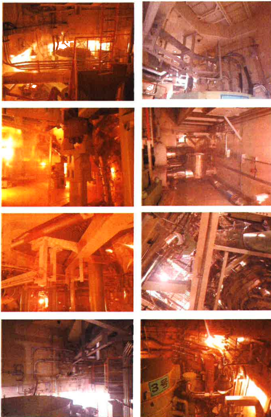
第 3-6-6 図 現場写真 (格納容器ループ室)
