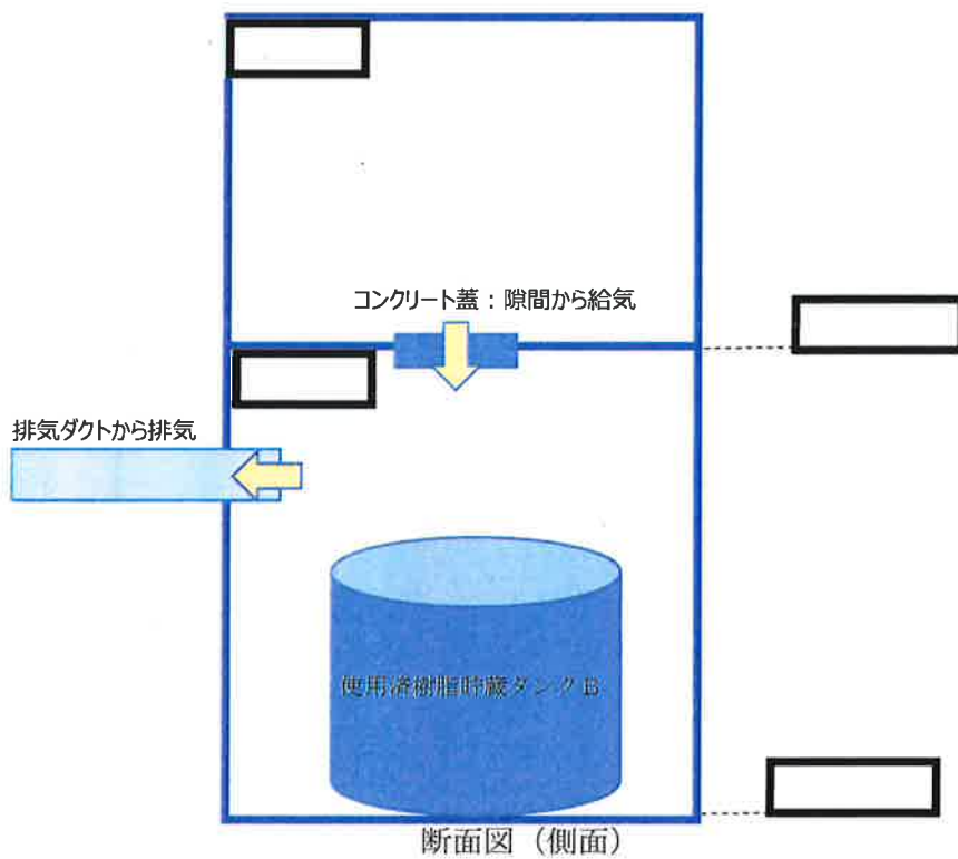
第 3-6-5-8-1 図 使用済樹脂貯蔵タンク室の空気の流れ (断面図)
