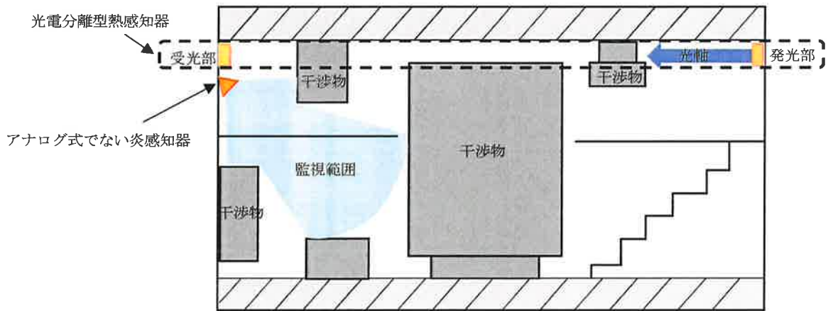
断面図
