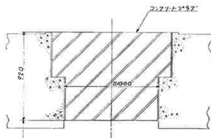
第 3-6-12 図 コンクリート蓋断面
