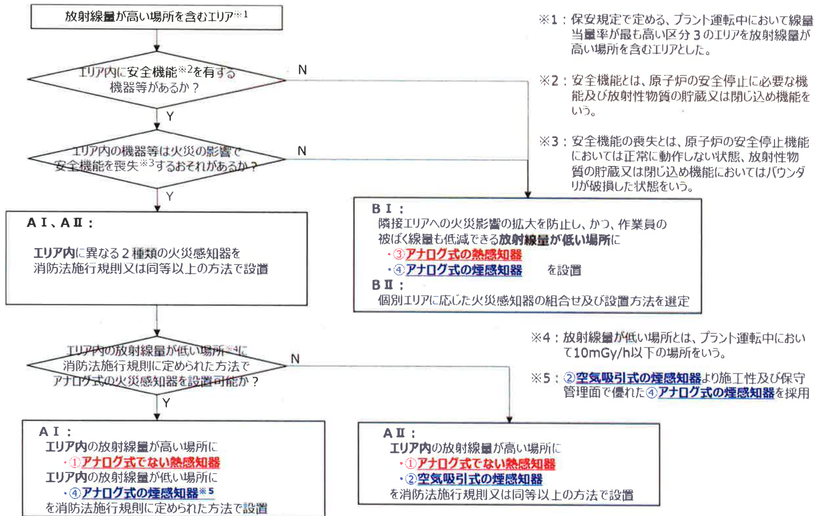
第 3-6-8 図 放射線量が高い場所を含むエリアの火災感知器設計フロー
