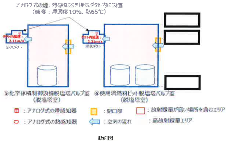
第 3-6-5-5-1 図 化学体積制御設備脱塩塔バルブ室、使用済燃料ピット脱塩塔バルブ室の空気の流れ (断面図)
