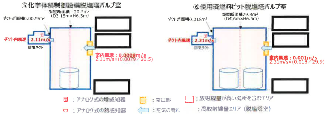
第 3-6-5-2 図 化学体積制御設備脱塩塔バルブ室及び使用済燃料ピット脱塩塔バルブ室の感知器配置図（脱塩塔室）
