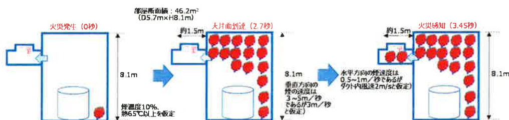
第3-6-5-8-4図 使用済樹脂貯蔵タンク室での火災発生時の空気の流れ
