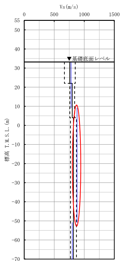
S 波速度
