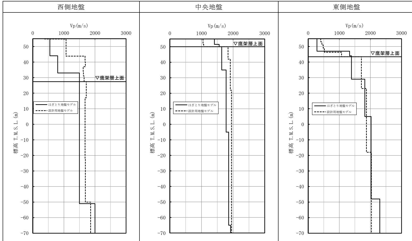
第 4.3-3 表(2) シミュレーション解析に用いた設計用地盤モデルとはぎとり地盤モデルの速度構造の比較 (P波速度)
