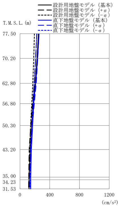
第 2.5.1.1-31 図 最大応答加速度 (鉛直方向 Sd-C1(UD))
