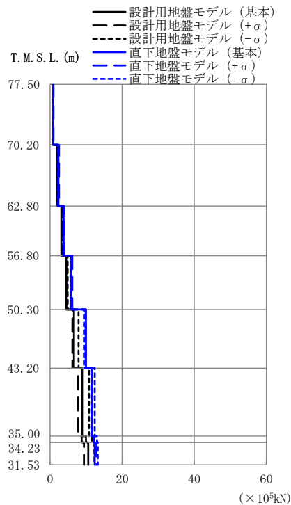
第 2.5.1.1-21 図 最大応答せん断力 (EW 方向 Sd-A(H))
