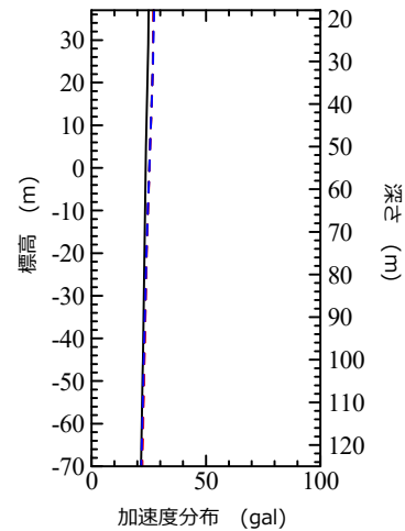
第 4.3-5 図(2) シミュレーション解析結果の 応答スペクトル図 (東側地盤, G.L.-18m) 及び最大加速度分布 (2011 年 3 月 11 日 2011 年東北地方太平洋沖地震)
