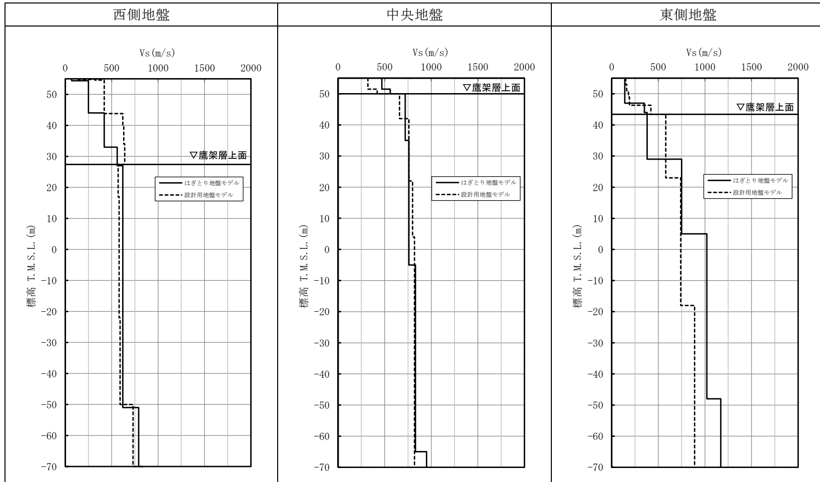
第 4.3-3 表(1) シミュレーション解析に用いた設計用地盤モデルとはぎとり地盤モデルの速度構造の比較 (S波速度)
