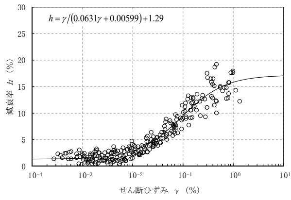
(b) 減衰特性
