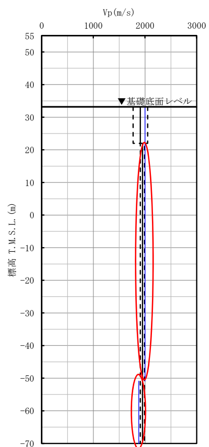
P 波速度
