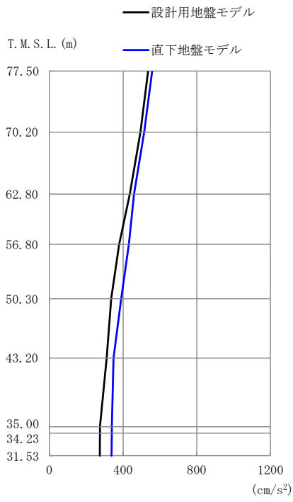
第 2.5.2.1-15 図 最大応答加速度 (鉛直方向 1.2×S s -C1(UD))
