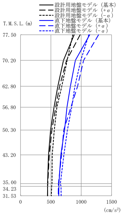
第 2.5.1.1-1 図 最大応答加速度 (NS 方向 S s -A(H))
