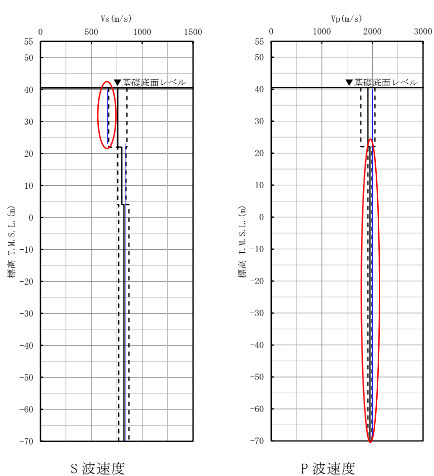
第 3.-6 図 主排気筒管理建屋における設計用地盤モデルと直下 PS 検層データとの速度構造の比較結果
