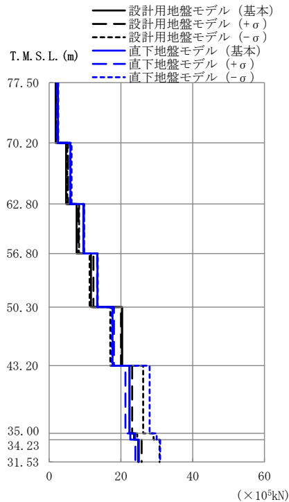
第 2.5.1.1-10 図 最大応答せん断力 (NS 方向 S s -C1 (NSEW))
