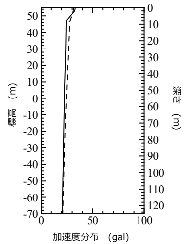
第 4.3-7 図(2) シミュレーション解析結果の 応答スペクトル図 (東側地盤, G.L.-11.6m) 及び最大加速度分布 (2011 年 3 月 11 日 2011 年東北地方太平洋沖地震)
