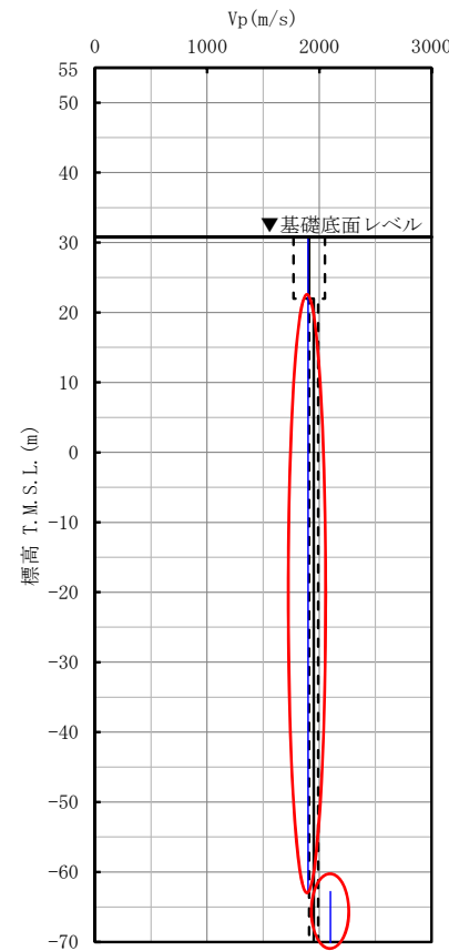
P 波速度
