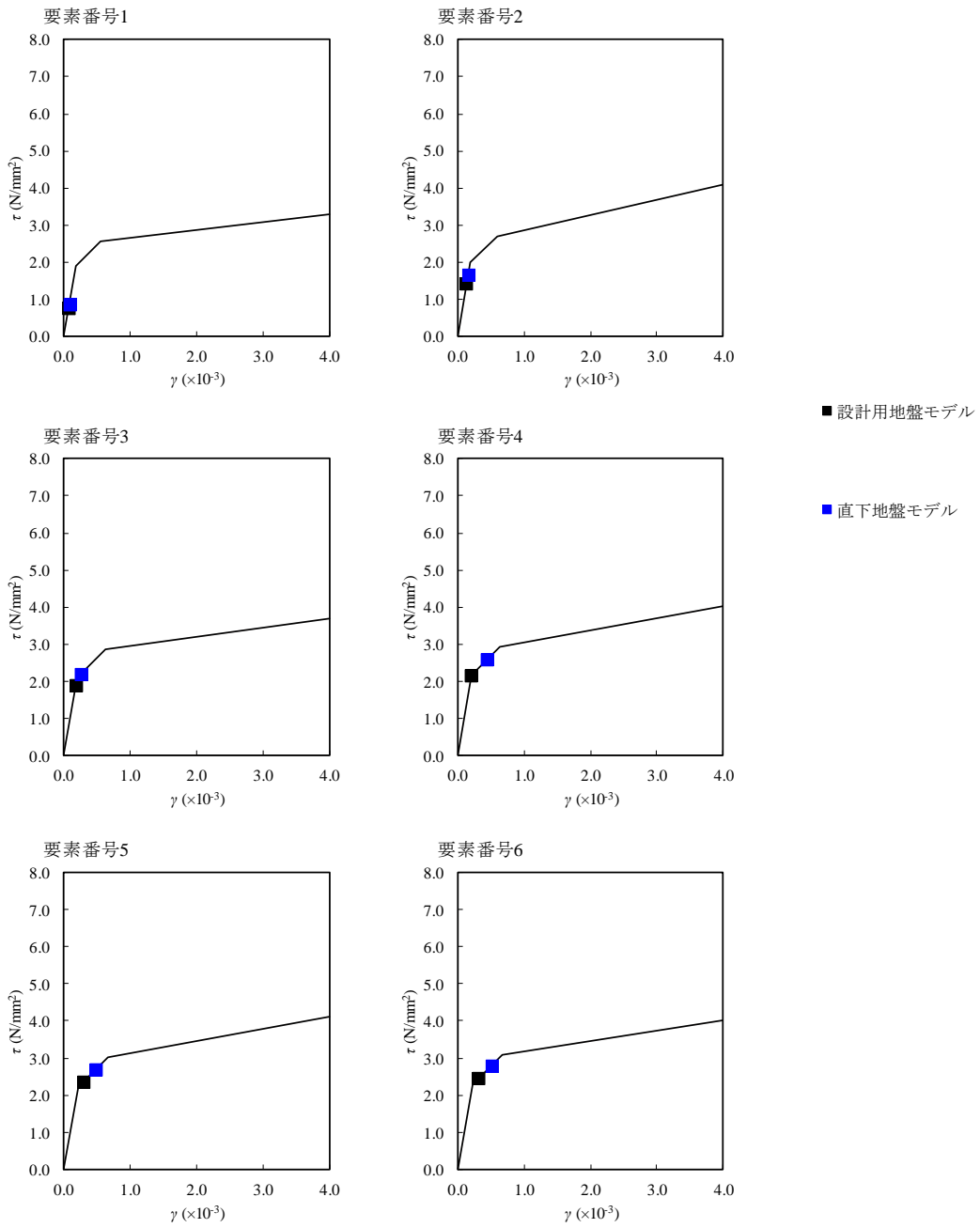
第 2.5.2.1-20 図 \tau - \gamma 関係と最大応答値 (EW 方向 1.2 \times S_s - C1 (NSEW))
