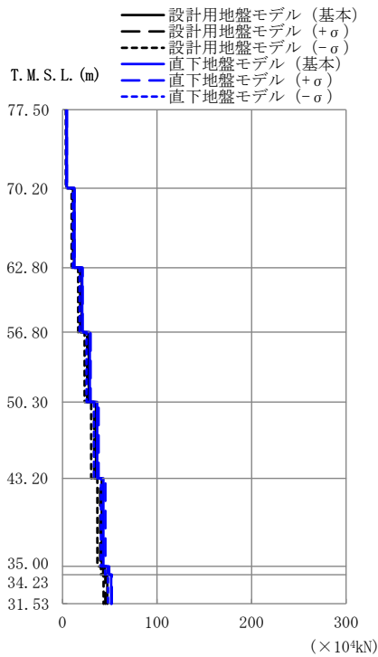
第 2.5.1.1-32 図 最大応答軸力 (鉛直方向 Sd-C1(UD))
