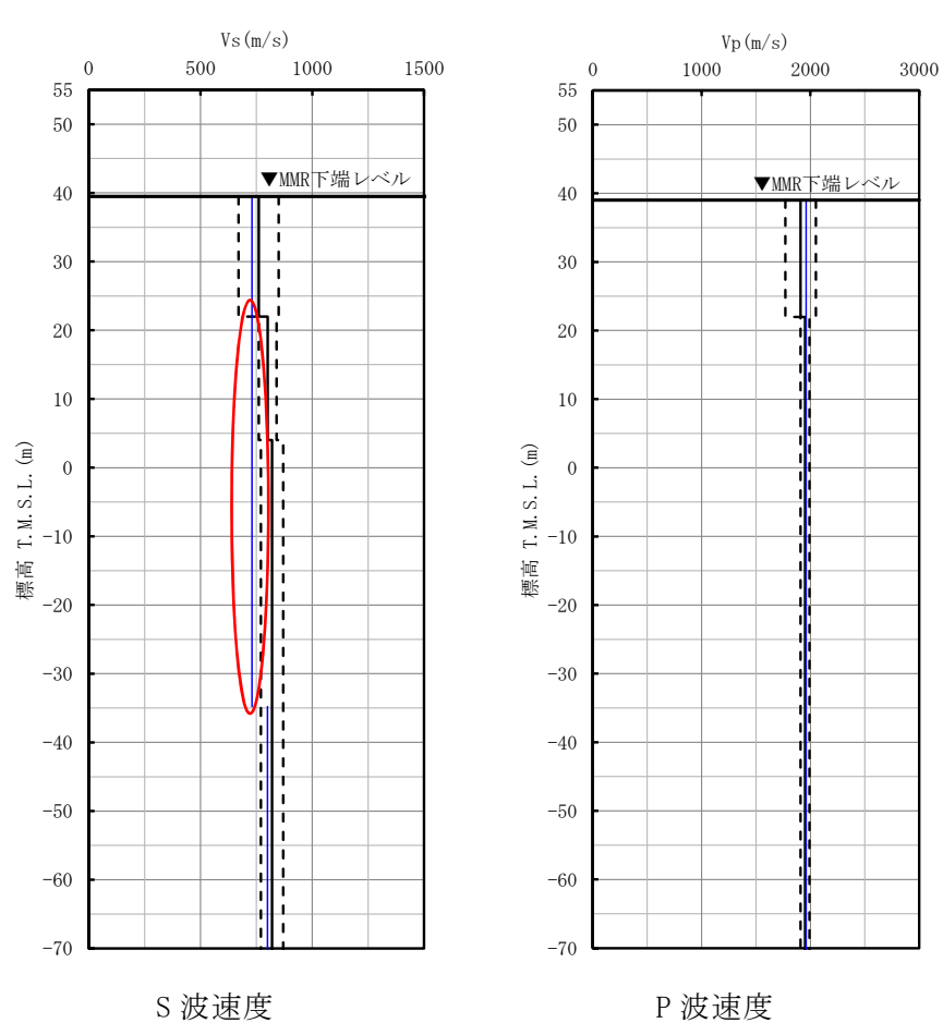
第 3.-18 図 非常用電源燃料タンク基礎における設計用地盤モデルと直下 PS 検層データとの速度構造の比較結果
