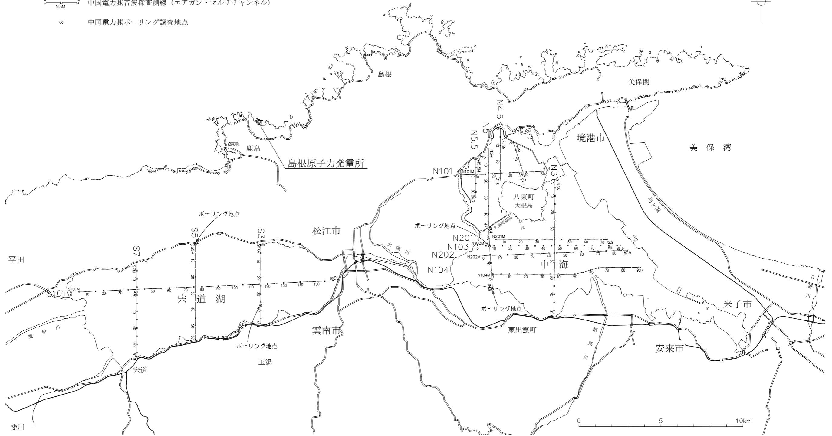
第3.2-5図(1) 宍道湖及び中海の音波探査測線図 (その1)
