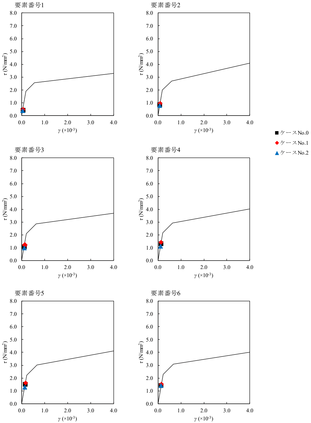
第3.2-17図 τ-γ関係と最大応答値 (Ss-B1, EW方向)
