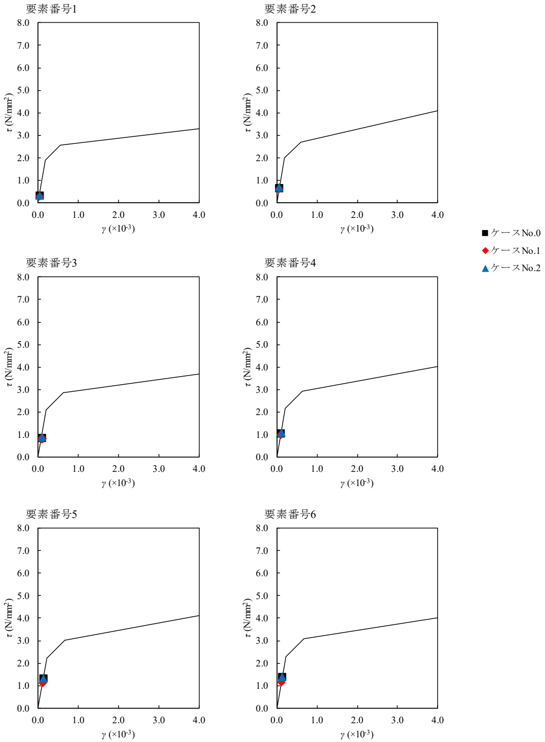
第 3.2-36 図 \tau - \gamma 関係と最大応答値 (Sd-C1, EW 方向)
