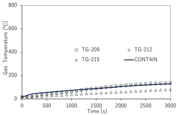
(b) ガス温度時刻歴変化・連通室
