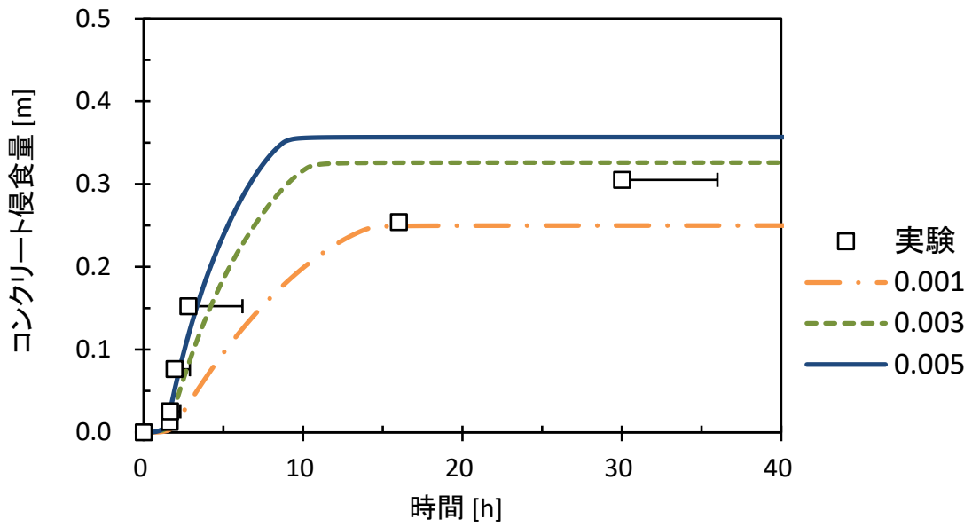
第 21 図 大規模ナトリウム-コンクリート反応実験 (LSC-1) におけるコンクリート侵食量 (FRACV=0.001, 0.003, 0.005 の感度解析)
