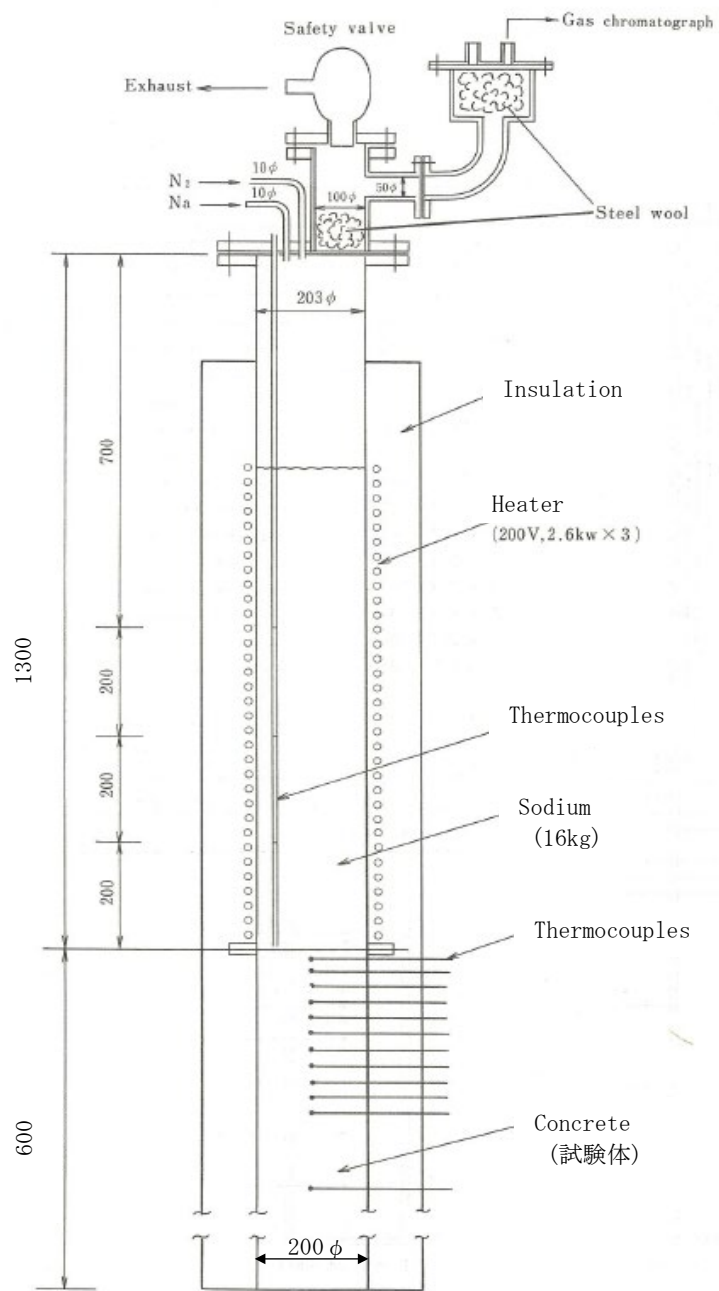
第 16 図 ナトリウム-コンクリート反応実験装置 (III-1M)
