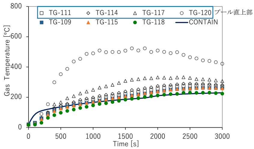
(a) ガス温度時刻歴変化・燃焼室
