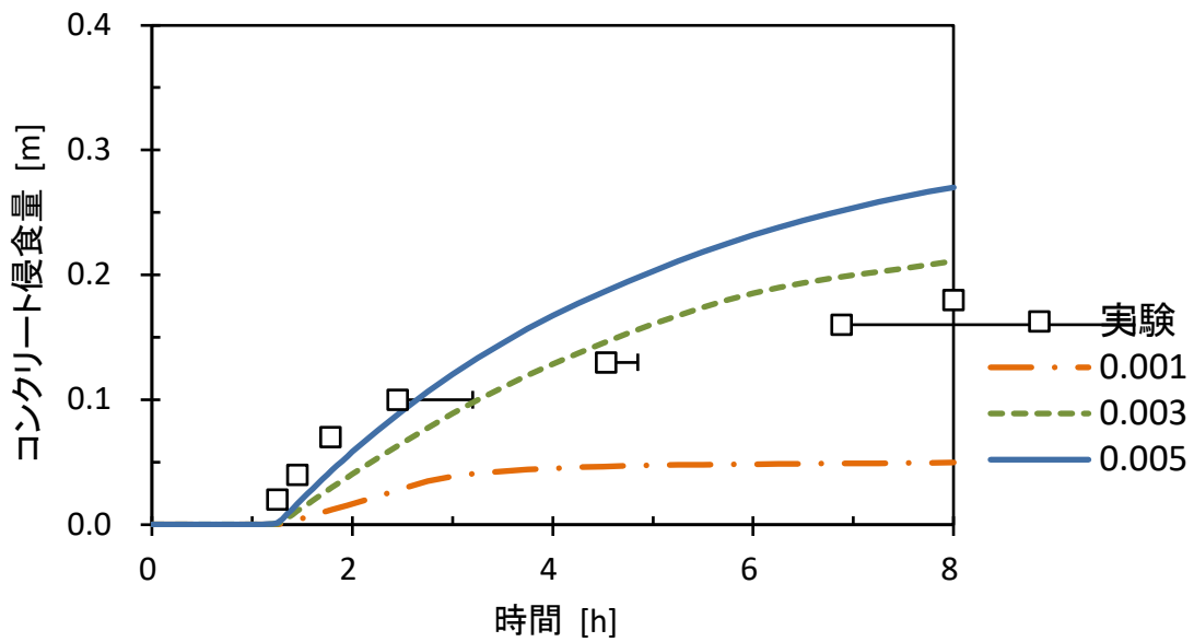
第 17 図 ナトリウム-コンクリート反応実験(Ⅲ-1M)におけるコンクリート侵食量 (FRACV=0.001, 0.003, 0.005 の感度解析)
