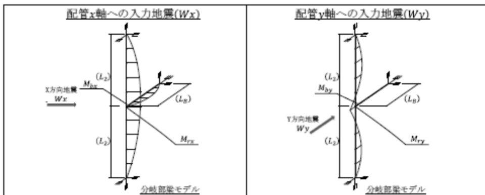
第3.4.2-6(3)図 配管（分岐部）モデル
