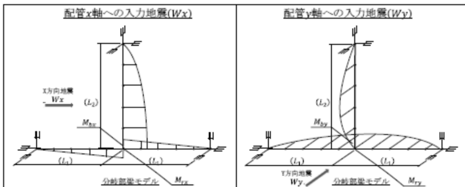
第3.4.2-6(2)図 配管（分岐部）モデル
