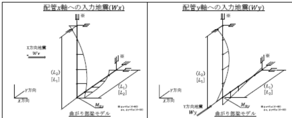
第3.4.2-4(2)図 配管（曲がり部）モデル
