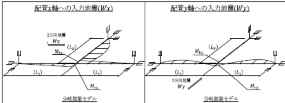
第3.4.2-6(1)図 配管（分岐部）モデル
