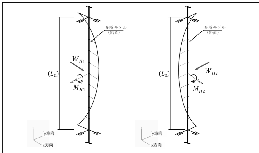
第3.4.2-2図 水平地震による鉛直配管の発生曲げ荷重概念図
