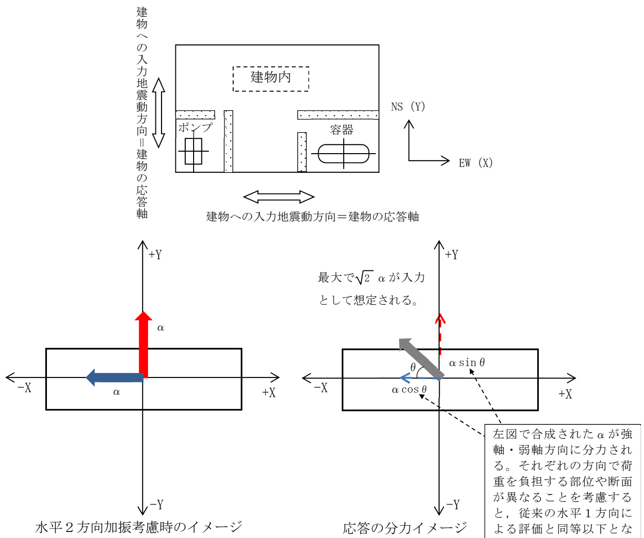
第 3.4.1-1 図 水平2方向同時加振時の応答イメージ
