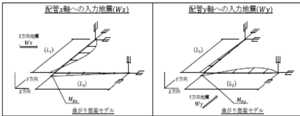
第3.4.2-4(1)図 配管（曲がり部）モデル
