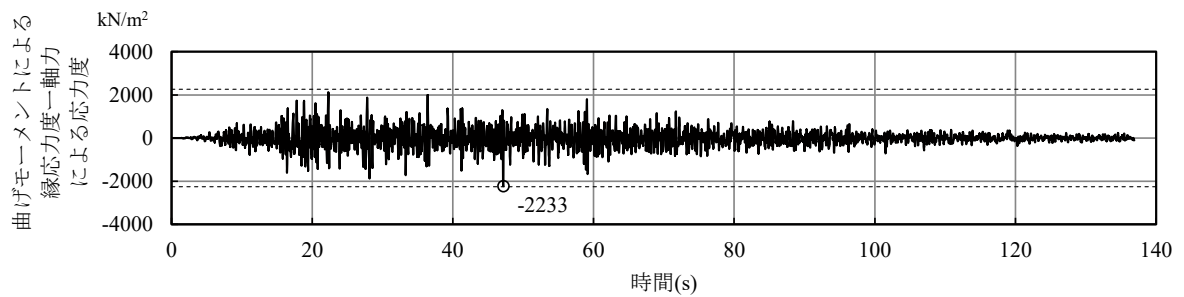
(b) 曲げモーメントによる縁応力度 (Sd-A) - 軸力による応力度 (Sd-A)
