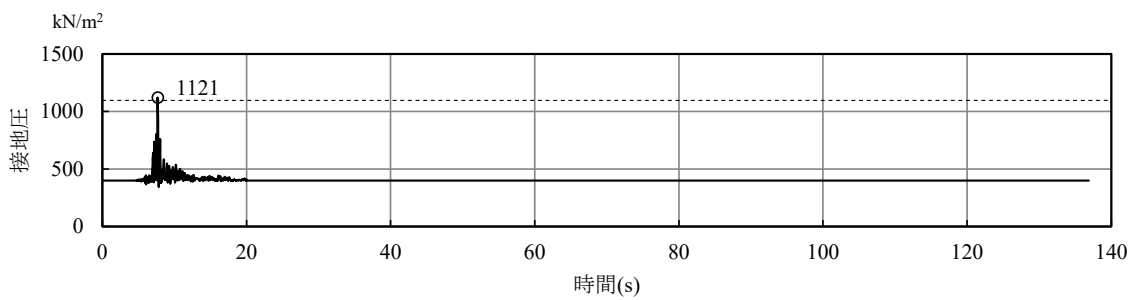
(a) 自重+EW 方向 (Ss-C1) +鉛直方向 (Ss-C1)
