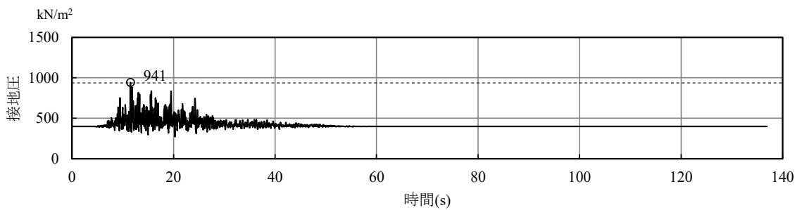
(a) 自重+EW 方向 (Ss-B5) +鉛直方向 (Ss-B5)
