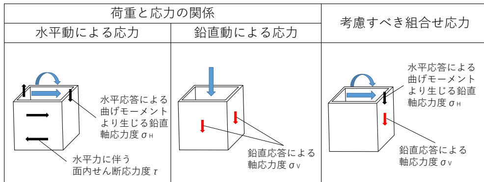
第 1.2-3 表 上部構造物の組合せ応力
