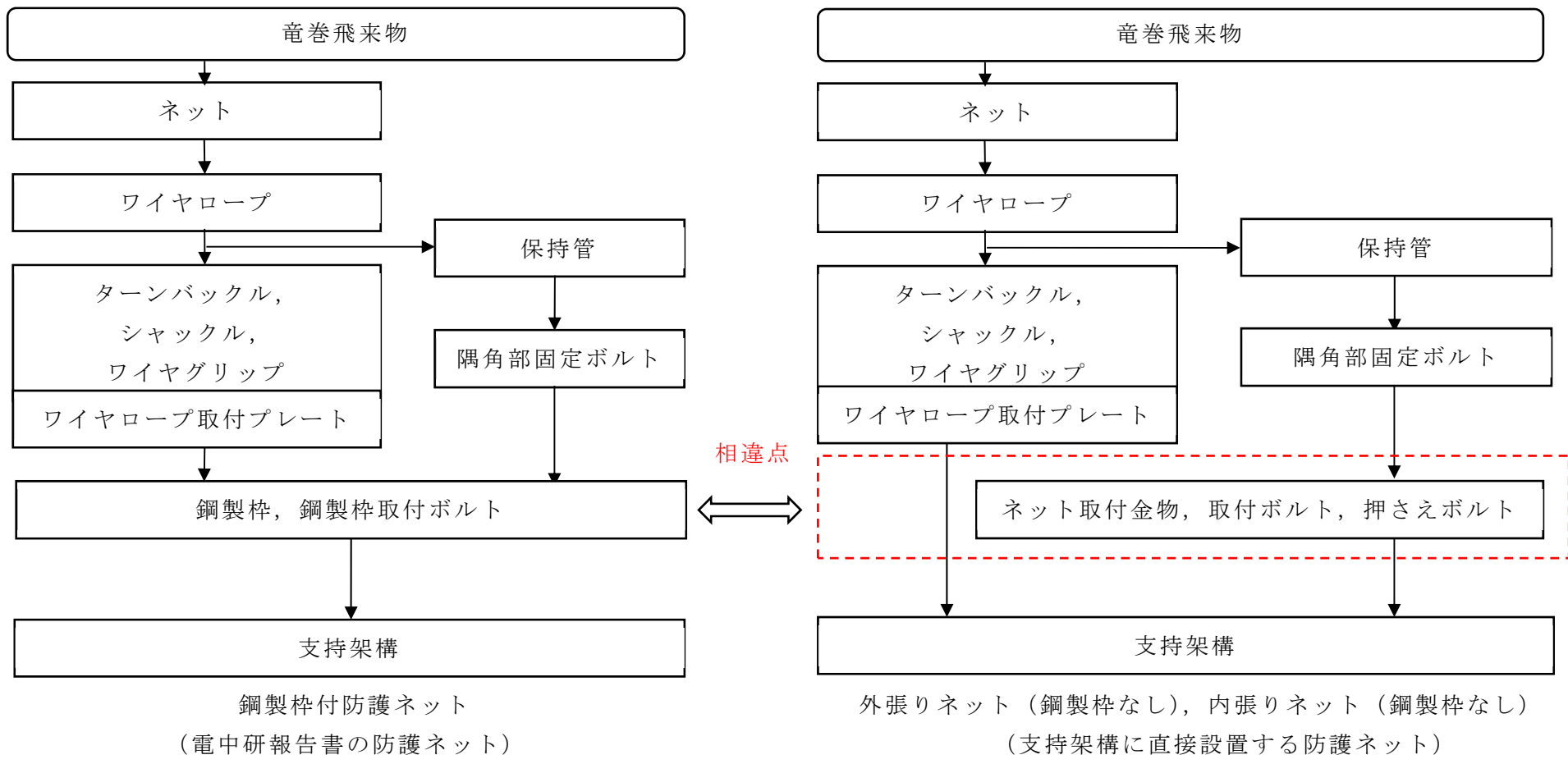
第5-4図 防護ネットの荷重伝達機構の比較
