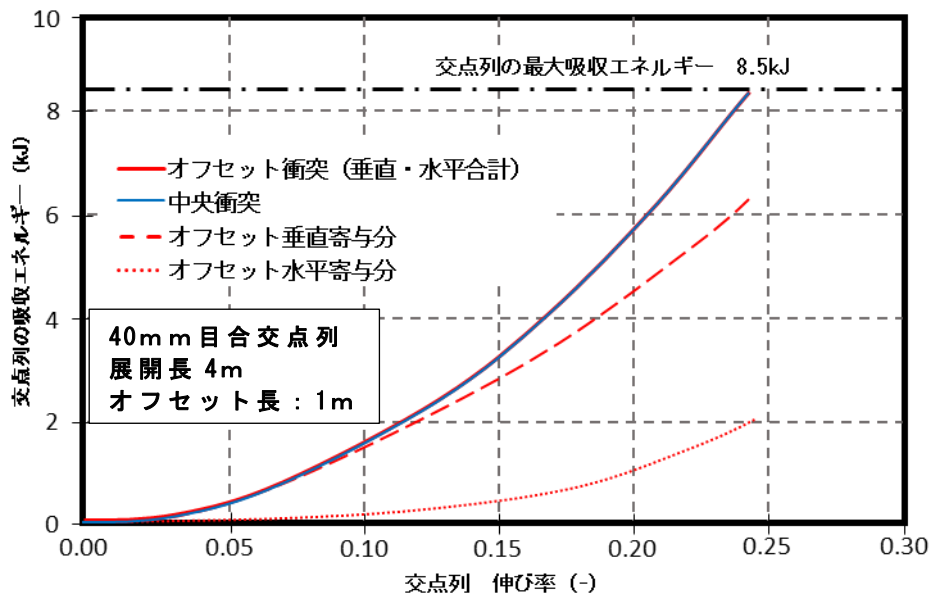
第2-6図 展開方向オフセット衝突と中央衝突のエネルギー比較（目合40mm）
