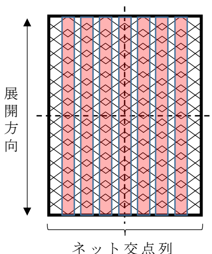
第 2-1 図 展開方向におけるネット交点列
