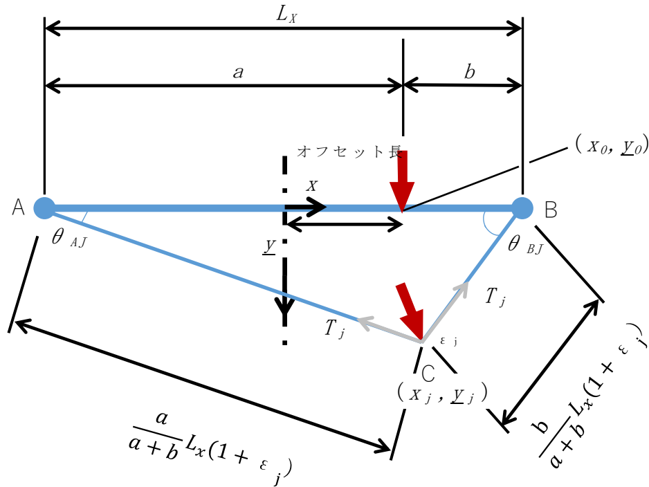
第2-4図 展開方向オフセット衝突の交点列変形状態の模式図
