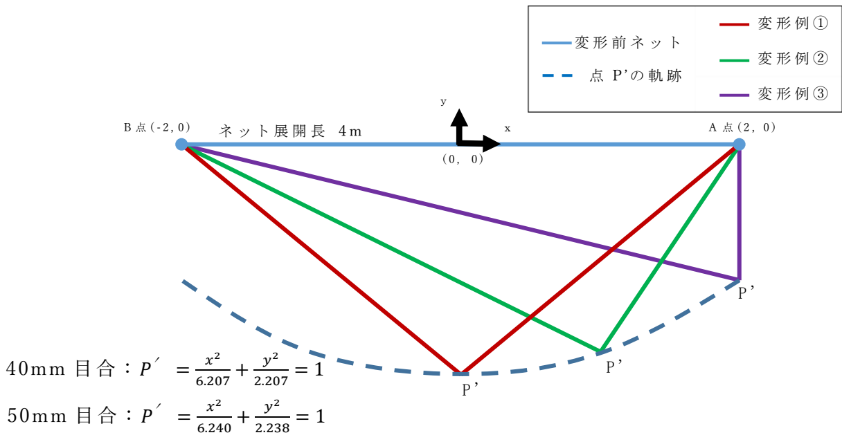
第 2 - 2 図 展開方向のネット交点列の衝突点 P' の軌跡
