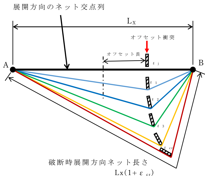
第2-3図 展開方向オフセット衝突時の展開方向のネット交点列の変位挙動図
