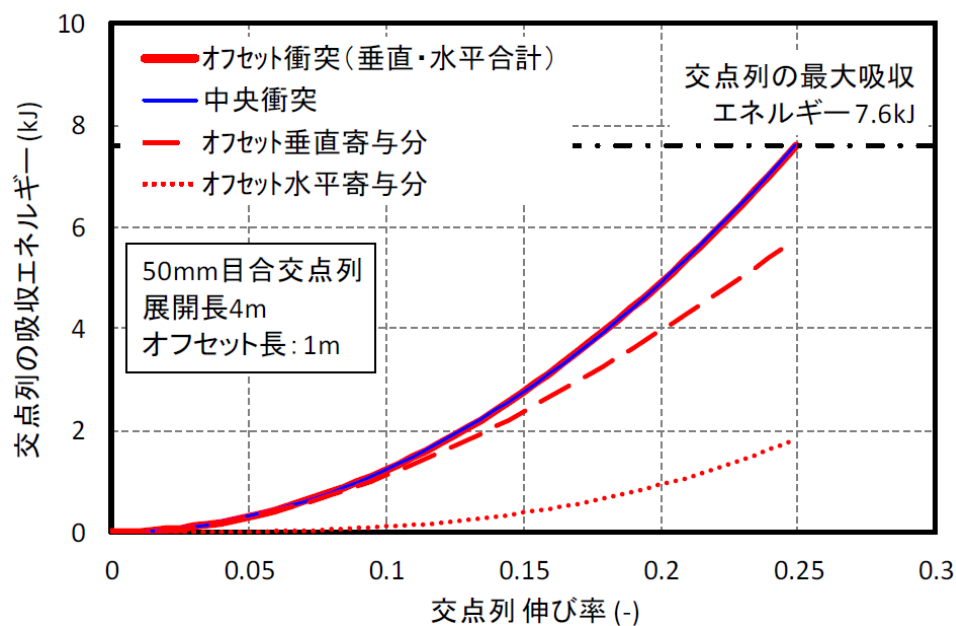
第 2-5 図 展開方向オフセット衝突と中央衝突のエネルギー比較 (目合 50mm)
