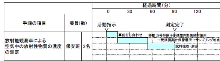
第 1.17.4 図 放射能観測車による空気中の放射性物質の濃度の測定のタイムチャート
