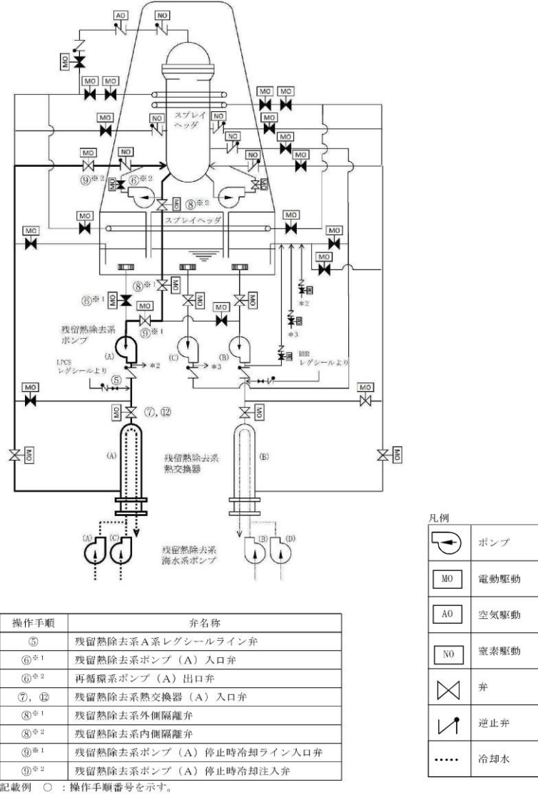
第 1. 4-27 図 残留熱除去系（原子炉停止時冷却系）電源復旧後の発電用原子炉からの除熱 概要図
