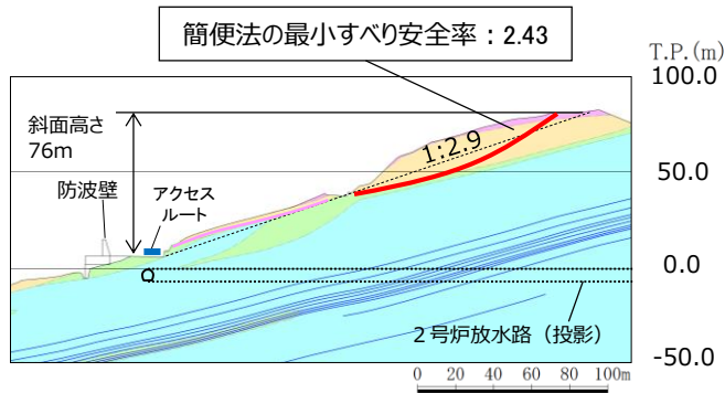
⑦—⑦' 断面
