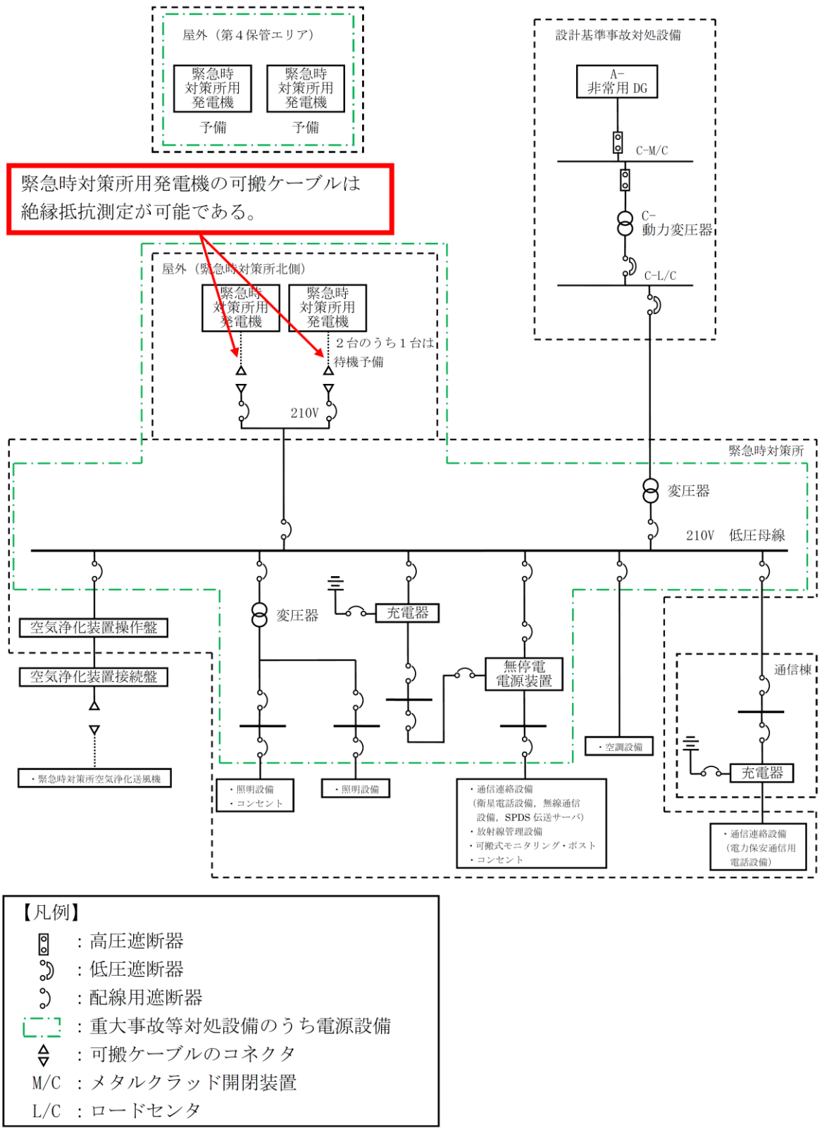
第 61-5-4 図 可搬ケーブル 試験系統図
