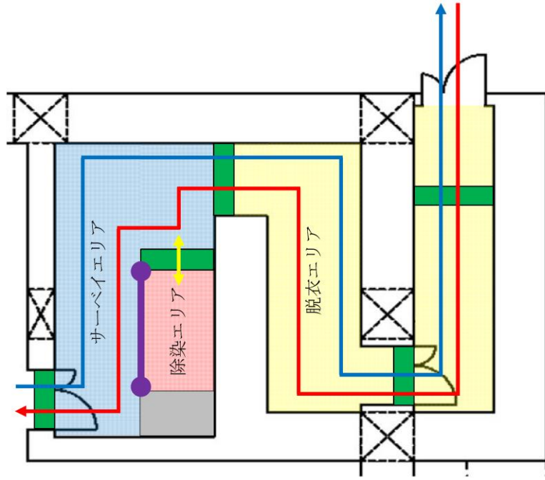
第3.3-1 図 緊急時対策所チェンジングエリア設営場所及び概略図
