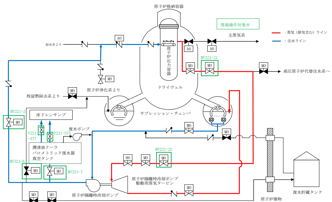
図4 原子炉隔離時冷却系 設備概要 (現場手動操作)
