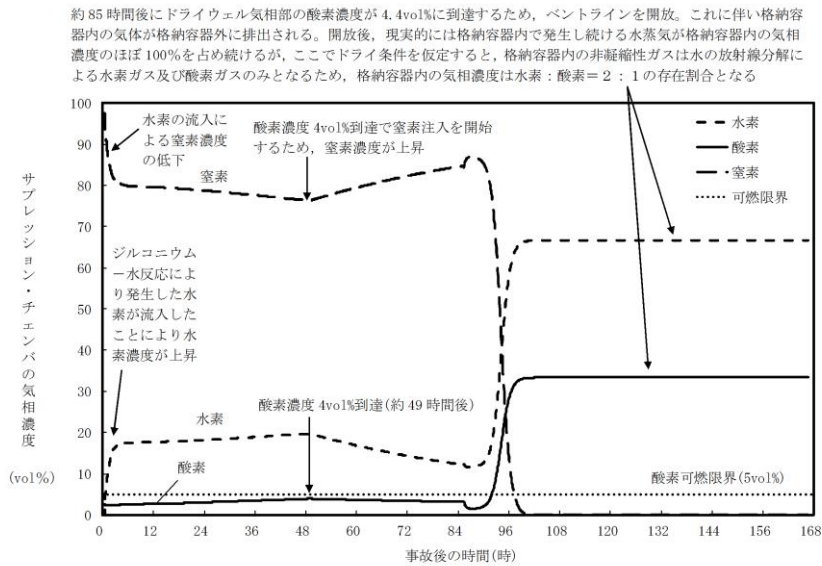
図2 「水素燃焼」において可燃性ガス濃度制御系の性能評価で使用しているG値を採用した場合のサブプレッション・チェンバの気相濃度の推移（ドライ条件）
