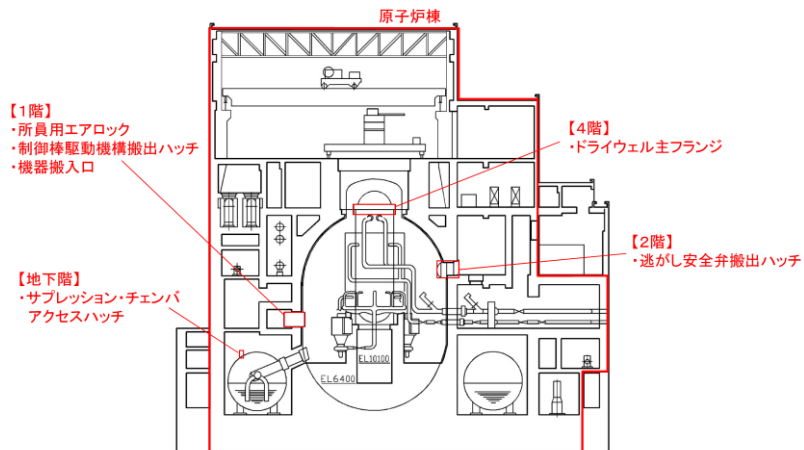
図 2.2.2-1 想定漏えい箇所
