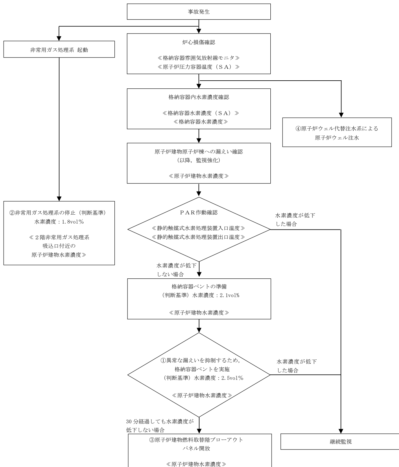
図 10 水素漏えい時の対策フロー
