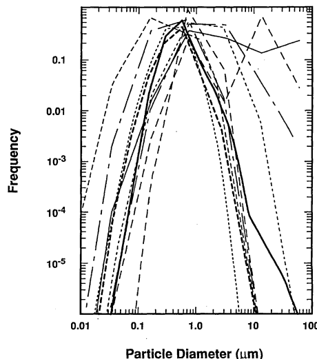
図2 格納容器内の粒子状物質の粒径分布 (NUREG/CR-5966より)
